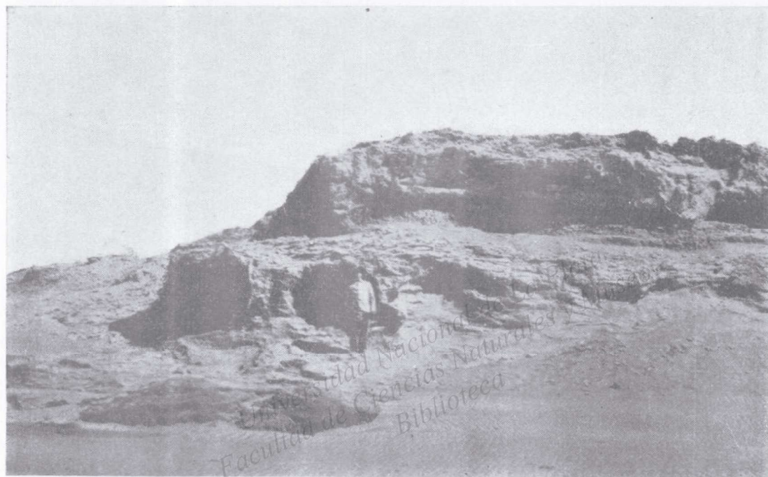
Fig. 5. — Barranca cortada en limos pampeanos (“Chapalmalense” y “Ensenadense”) en la costa atlántica cerca de Miramar.
