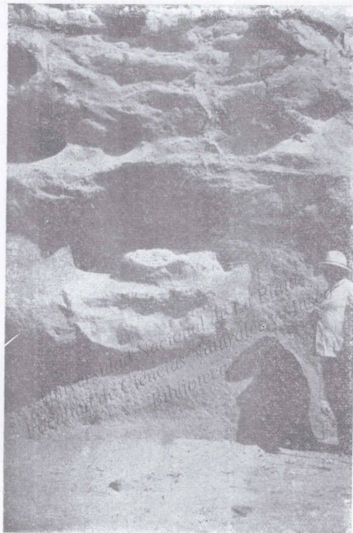
Fig. 7. — Superficie del Chapalmalense expuesta a la deflación en los acantilados marinos de Miramar.
