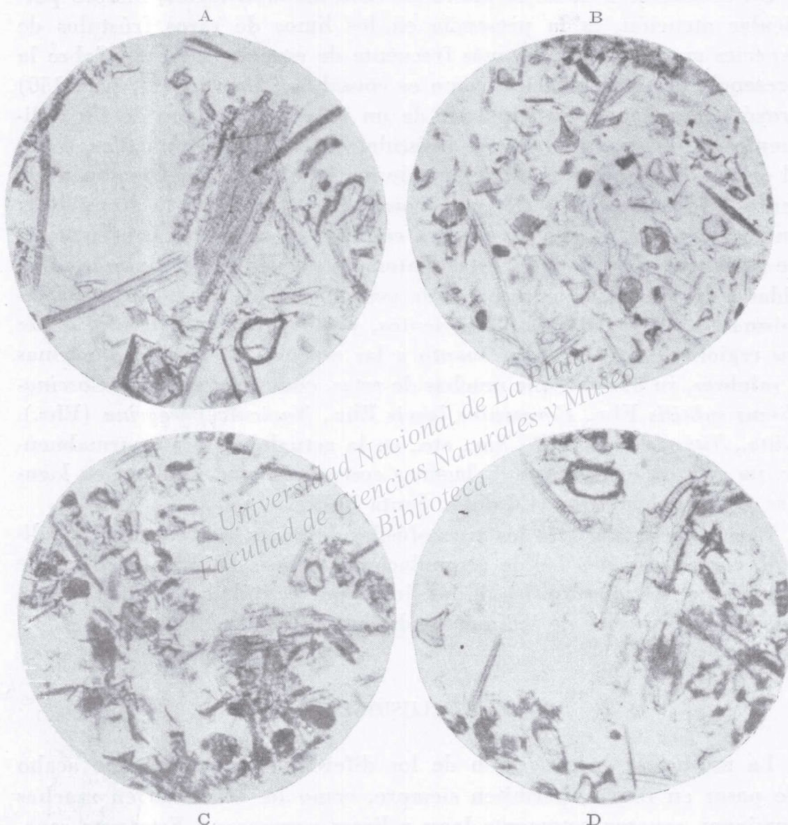
Fig. 24. — Residuo insoluble de limos pampeanos. — Células síliceas de gramíneas, espículas de esponjas, diatomeas, etc., del "Prebelgranense" de Miramar ("Ensenadense" de Ameghino). — A, x 250; B, x 100; C, x 75; D, x 150.
