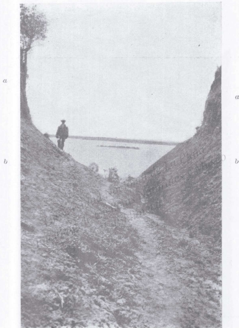
Fig. 9. — Parte superior de la barranca del borde izquierdo del río Paraná en los alrededores de la ciudad de Paraná: a , loess; b , limo.
