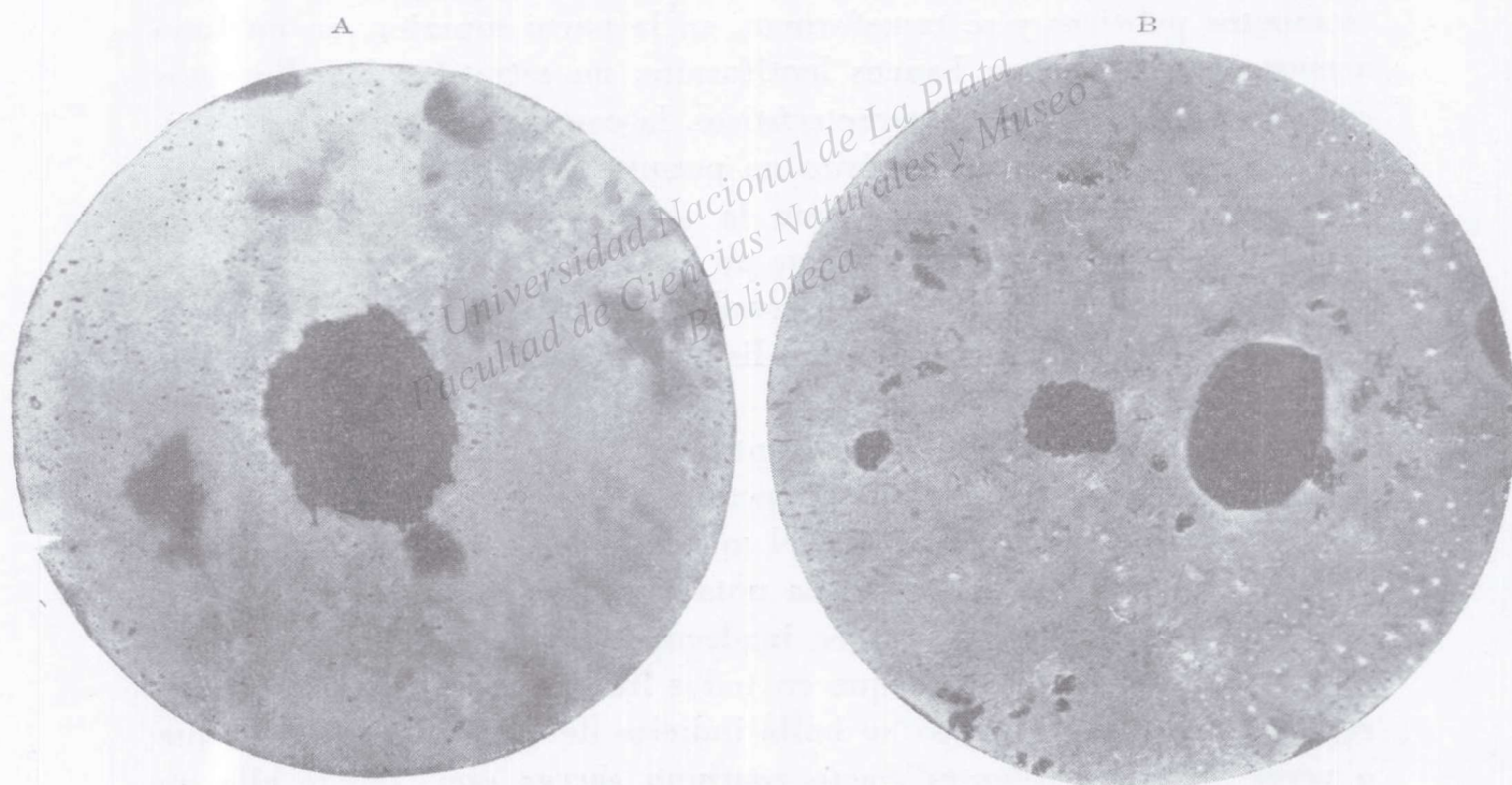
Fig. 1. — Esferulitas del loess pampeano “bonaerense” de los alrededores de Paraná. A y B \times 100 .
