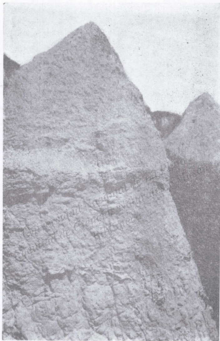
Fig. 10. — Pirámides de erosión sobre limo pampeano. Paraná, en proximidad de Parque Urquiza.
