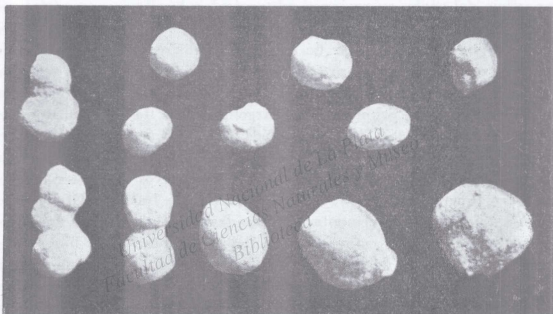
Fig. 18. — Tosquillas nodulares del loess pampeano —del "Bonaerense" de Santo Tomé (Santa Fe). Tamaño natural.
