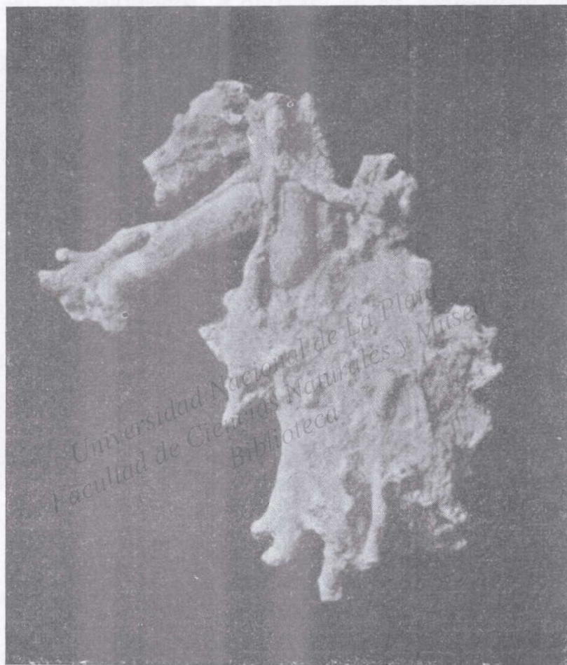
Fig. 20. — Tosquilla calcárea de limos pampeanos — del "Lujanense" de Esperanza (Santa Fe).
