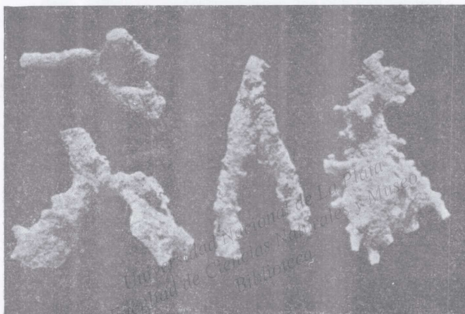
Fig. 19. — Tosquillas calcáreas de limos pampeanos — del "Ensenaden- se" de Santo Tomé (Santa Fe).
