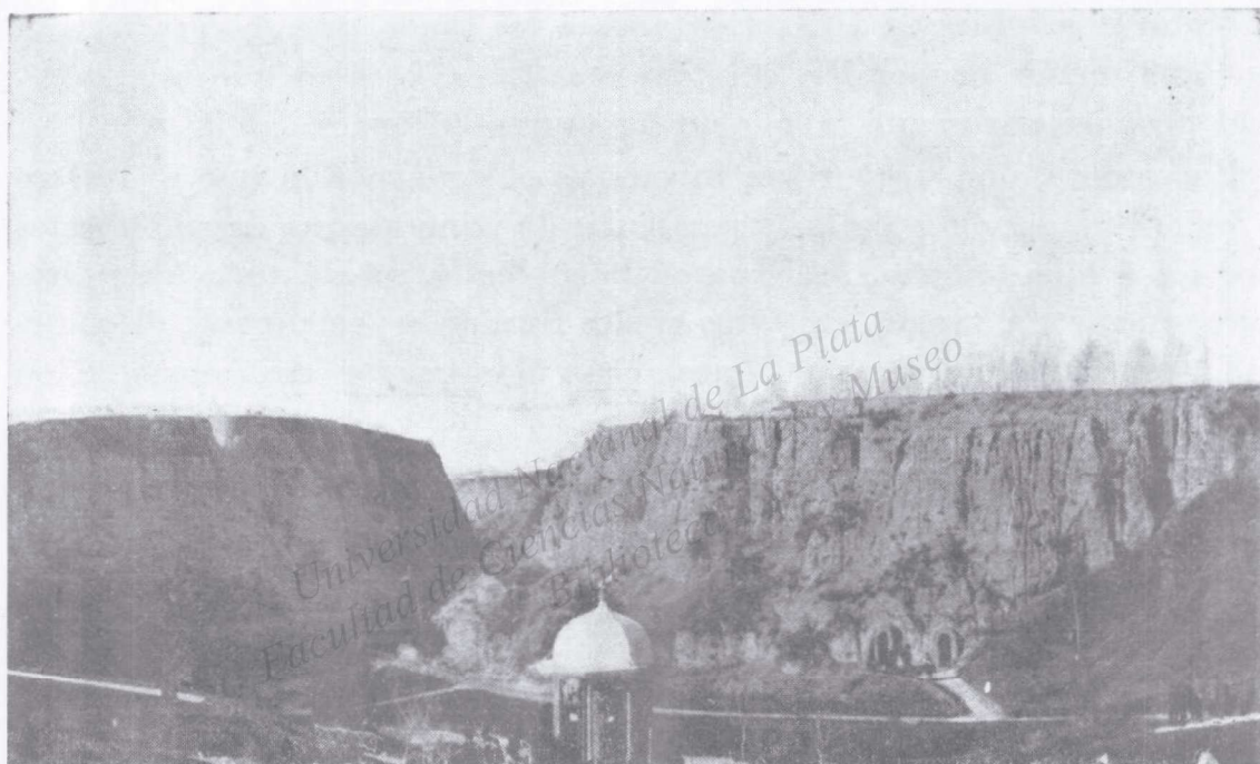
Fig. 4. — Barrancas cortadas en loess pampeano. — Terraza superior (meseta) del valle del río Primero en Córdoba (Jardín Zoológico).
