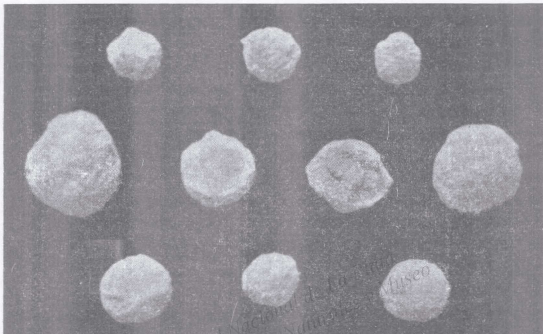
Fig. 2. — Bolillas subpisolíticas de limo pampeano. — Tamaño natural.
