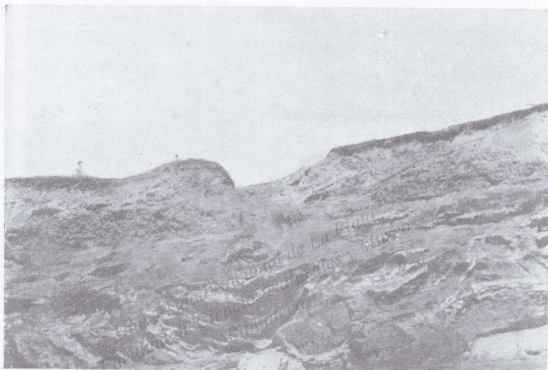
Fig. 6. — Limo pampeano endurecido y expuesto a las acciones meteóricas. Barranca de la costa cerca de Miramar.
