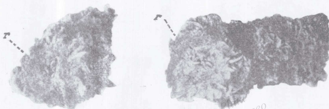
Fig. 22. — Tosquillas de yeso con restos de raíces (r) en el canalículo axial — del limo querandinense en el arroyo de las Brusquitas. — Algo ampliadas.
