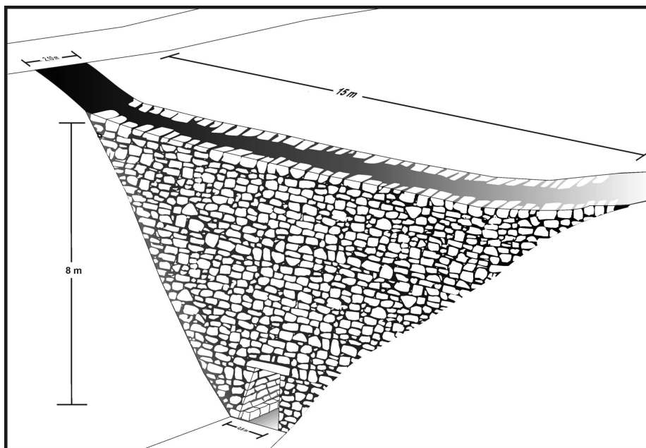
▲ Fig. 6. Croquis del puente de Ñoquera.
