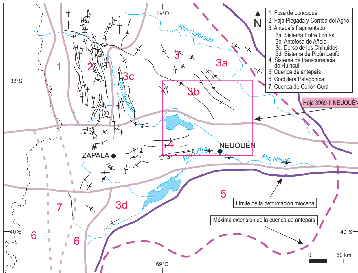
Figura 7. Situación de la Hoja 3969-II, Neuquén en el contexto de las unidades morfoestructurales de la cuenca Neuquina. Adaptado de Mosquera y Ramos (2005).
