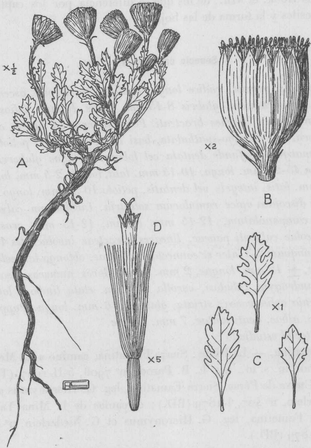
Fig. 2. — Senecio cremnicola Cabr. (Tipo) : A, planta; B, capitulo; C, hojas; D, flor
