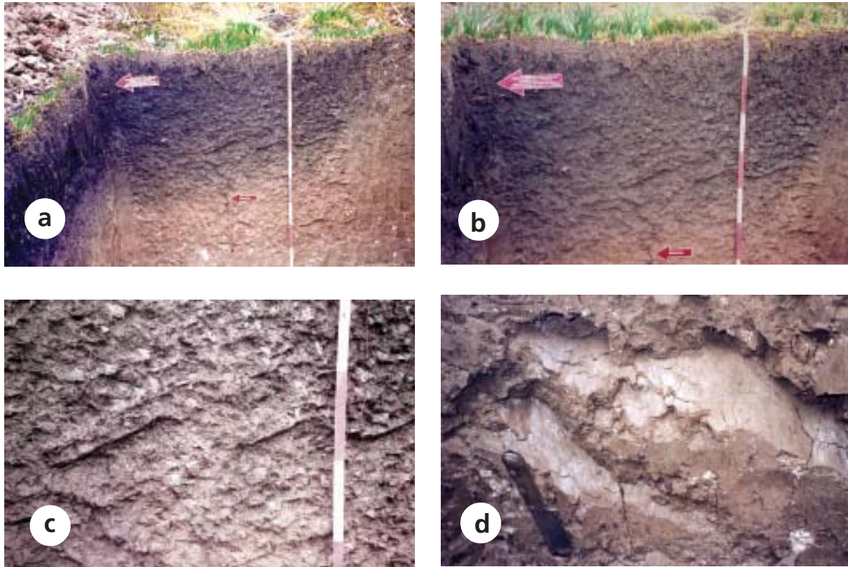
Figura 5.4. Morfología típica de Vertisoles fuertemente desarrollados, provincia de Entre Ríos: a) Serie San Gustavo en el bajo del gilgai, b) zona con superficies de deslizamiento, c) detalle de la zona con superficies de deslizamiento entrecruzadas, d) detalle de superficie de deslizamiento.
