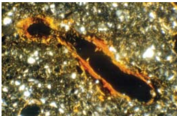
Figura 3.12. Revestimientos texturales arcillosos en suelos actuales en horizonte BC2 (120-147 cm) de un Argialbol. Partido de Brandsen, provincia de Buenos Aires. 30X.
