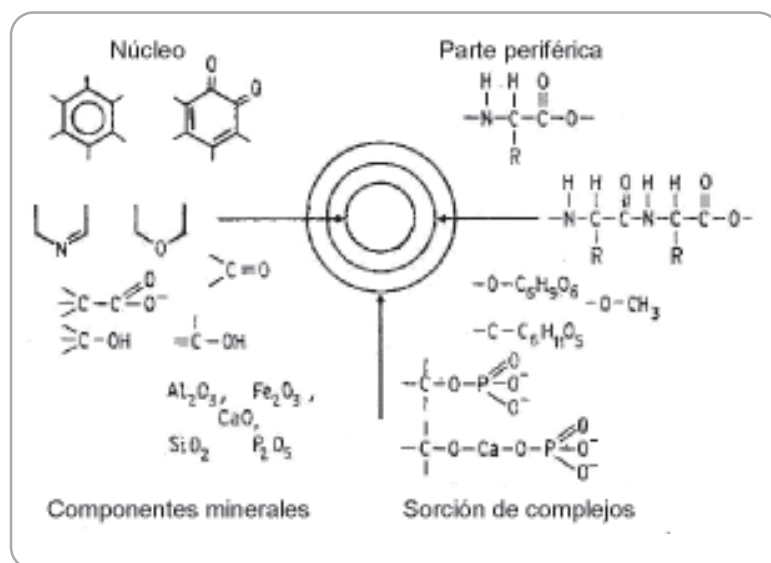
Figura 2.4. Esquema estructural de las sustancias húmicas según Mistetskii y Loginov (1959).
