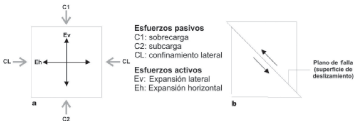
Figura 5.10. Modelo mecánico de formación de superficies de deslizamiento en un sistema confinado. a) Componentes de los esfuerzos asociados. b) Orientación de los planos de corte a 45° respecto al esfuerzo principal. Modificado de Wilding y Tessier, 1988.
