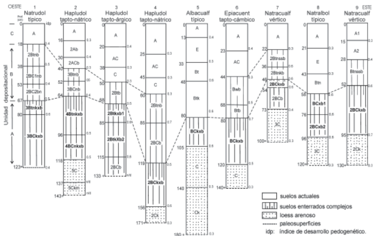
Figura 3.10: Distribución regional de paleosuelos. Área de interdunas. Pampa Arenosa, provincia de Buenos Aires. 1-2 Crlos Tejedor; 4-5-6 Saladillo; 7-8-9 Roque Pérez. Modificado de Imbellone et al.; 2005.
