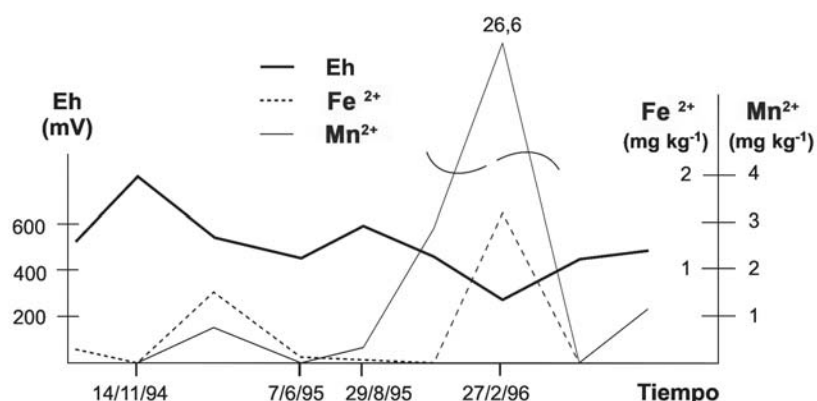
Figura 4.6. Relación de Eh con \text{Fe}^{2+} y \text{Mn}^{2+} . Horizonte A. Pedón 2.
