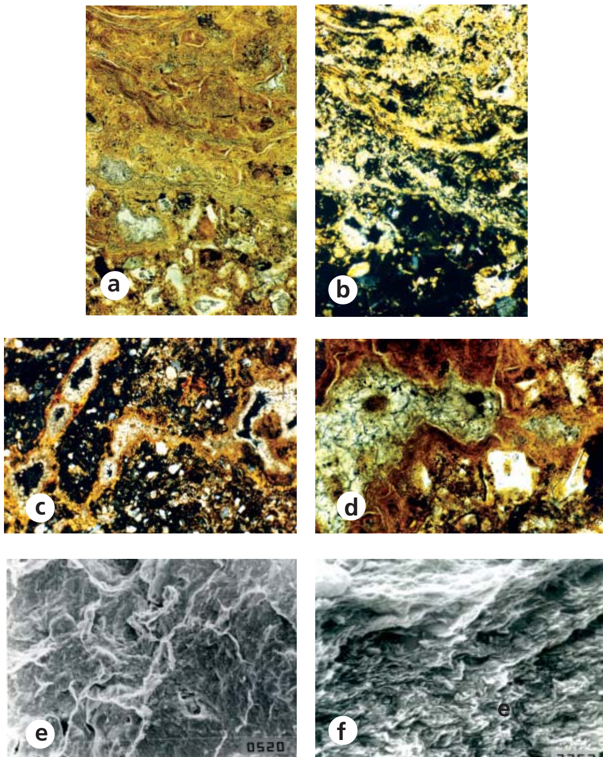
Figura 3.11. Micromorfología de fragipanes, Pampa Arenosa, provincia de Buenos Aires. a) horizonte 2Btb ilimerizado y carbonatado, microscopía óptica, 50X, b) ídem anterior, con analizador, 50X, c) horizonte 2Btb ilimerizado y carbonatado en vacíos de conducción, microscopía óptica, 30X, d) detalle de c) mostrando revestimientos arcillosos y calcita esparítica obliterando vacíos de conducción, 80X, e) vista superficial de un agregado, microscopía electrónica de barrido, 1500X, f) vista lateral del fragipán mostrando ordenamiento subparalelo del material, microscopía electrónica de barrido, 1000X.
