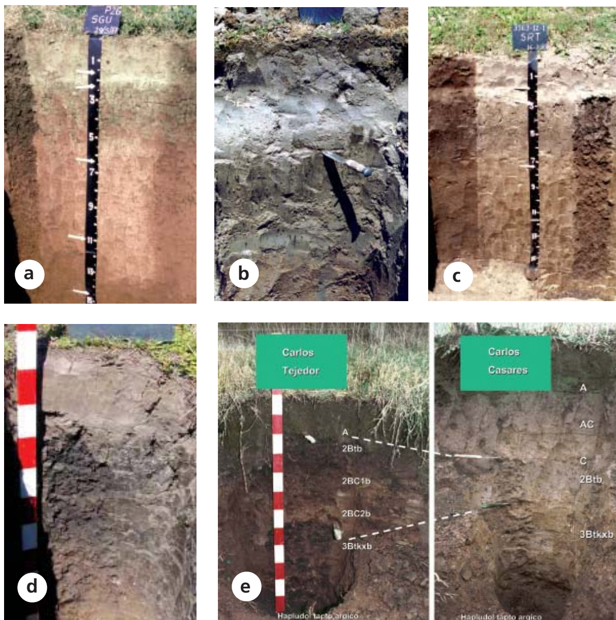
Figura 3.1. Suelos con proceso de ilimerización de la Región Pampeana. a) Argialbol típico. Serie San Guillermo, provincia de Santa Fe, b) Argialbol típico. Partido de La Plata, provincia de Buenos Aires, c) Albacualf típico. provincia de Santa Fe, d) Argiudol vértico. Partido de La Plata, provincia de Buenos Aires, e) Hapludoles tapto-árgicos de la Pampa Arenosa, provincia de Buenos Aires, f) Grandes Grupos de suelos con ilimerización.
