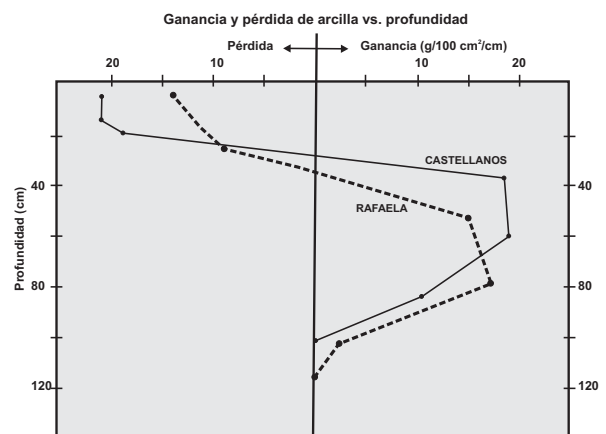
Figura 3.13. Ganancias y pérdidas de arcilla. Argiudol típico (Serie Rafaela), Argialbol típico. (Serie Castellanos). Panigatti, 1980.
