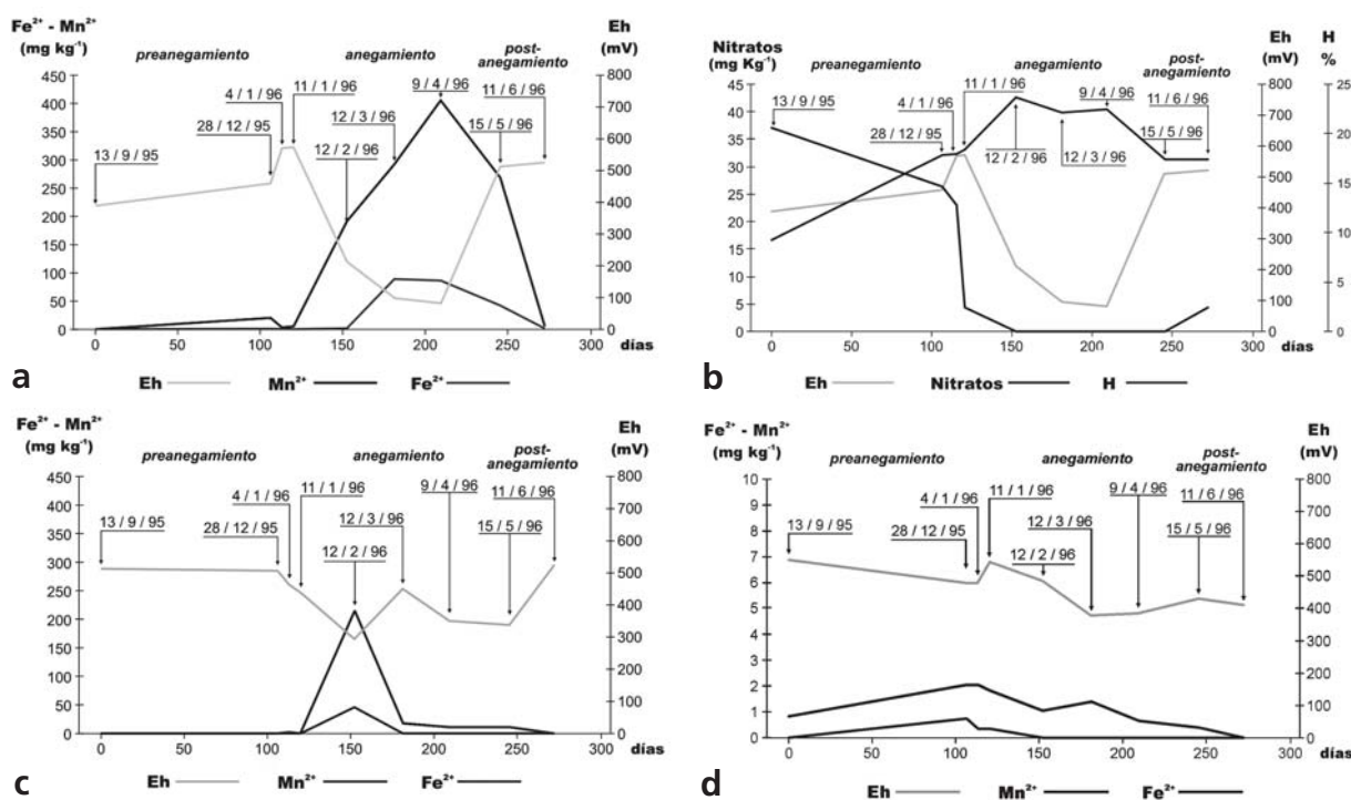
Figura 4.11. Evolución de variables hidromórficas en suelos sistematizados para cultivo de arroz, en distintos etapas del cultivo, a) Eh, Fe 2+ y Mn 2+ , horizonte Ap sembrado; b) Eh, nitratos y humedad, horizonte Ap sembrado; c) Eh, Fe 2+ y Mn 2+ , horizonte BA sembrado; d) Eh, Fe 2+ y Mn 2+ , horizonte Ap testigo.
