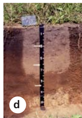
Figura 3.15. Suelos de una climosecuencia regional. a) Argiudol típico (Serie Villa Trinidad), b) Argiudol típico (Serie Colonia Mackinlay), c) Hapludol típico (Serie Colonia Alpina), d) Hapludol éntico (Serie Dos Provincias).
