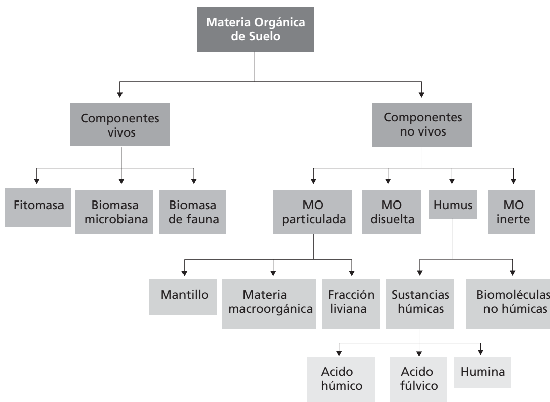
Figura 2.2. Componentes de la materia orgánica.
