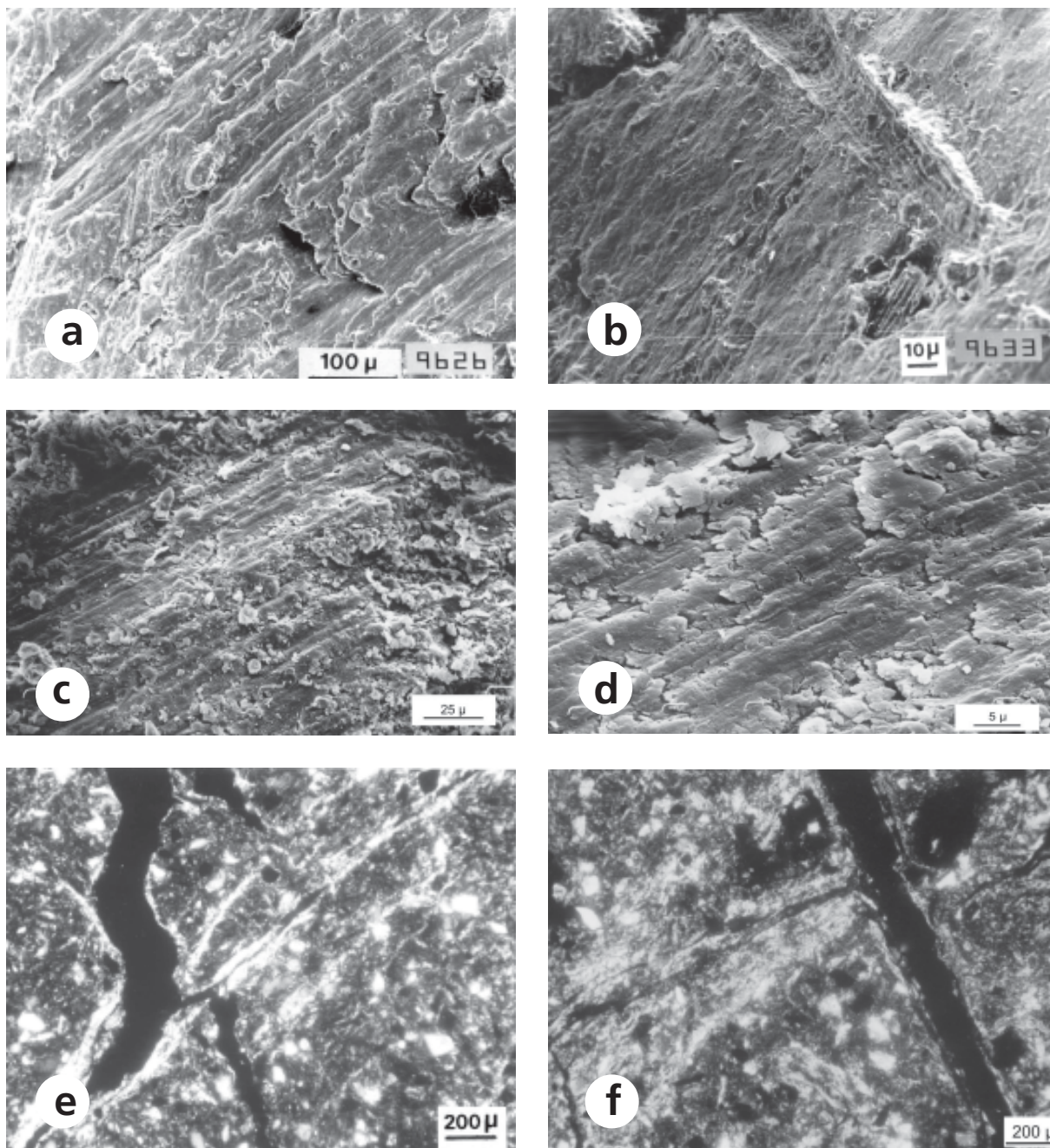
Figura 5.13 Rasgos micromorfológicos de suelos de la provincia de Buenos Aires. Superficies de deslizamiento y rasgos de matriz del suelo. Microscopía electrónica de barrido: Albaculf vértico a) horizonte Btss2 (76-125 cm) X 200; b) impronta de raíz X 750. Natracuert c) horizonte Bsg2 (26-58 cm), X500; d) detalle X 2000. Imbellone y Giménez, 1990. Microscopía óptica. Albaculf vértico, horizonte Btss2 (76-125 cm) X 30. e), f), g) fábrica de birrefringencia estriada con fisuras angulares; h) horizonte Bckss (125-148 cm) X 30 cavidades mamelonares orientadas, aisladas e intercomunicadas, rodeadas por argillanes finos. Imbellone, 1980.
