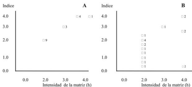
Figura 4.13. Relación entre el índice y la intensidad de la matriz para los horizontes: a) Bt y Bw de los Udoles y b) para los horizontes Bt y Bw de los Alboles, Acuoles y Acualfes. (Los números arábigos representan el número de horizontes considerados)
