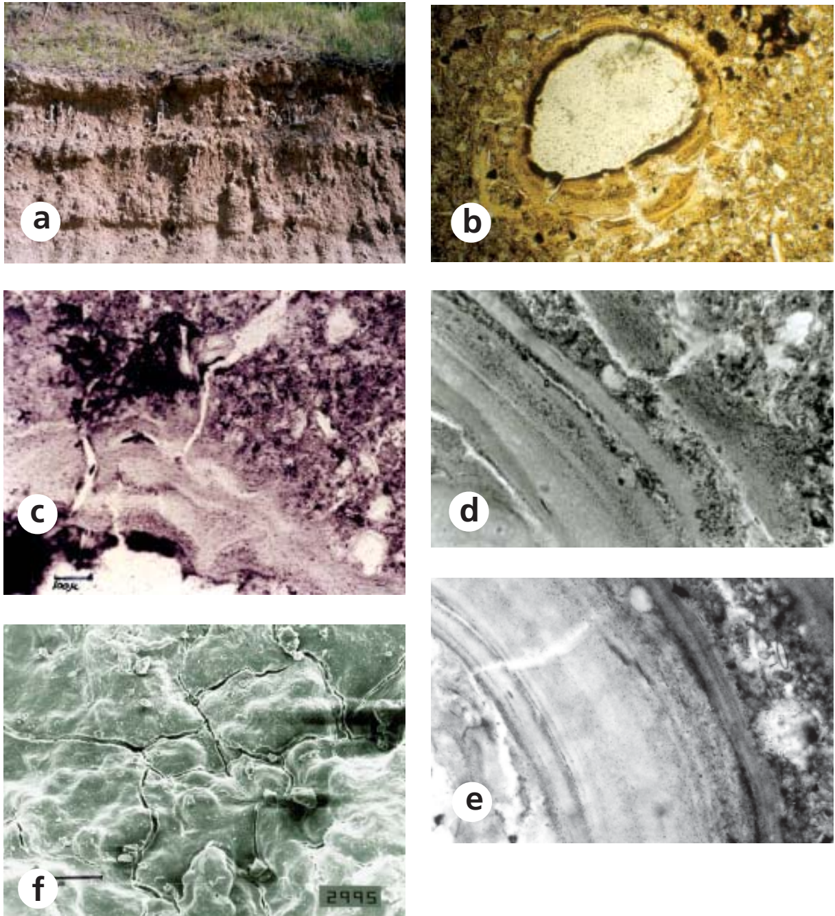
Figura 3.9. a) Suelos profundamente enterrados. Cantera de Hernández. Partido de La Plata, provincia de Buenos Aires, b) y c) revestimientos compuestos texturales y amorfos, microscopía óptica, d) y e) revestimientos texturales de limo y arcilla, microscopía óptica (nótese diatomea en banda limosa en e), f) revestimiento grueso de arcilla, microscopía electrónica de barrido. Aumentos: b) 30X, c) y d) 50X, e) 80X, f) 1000X.
