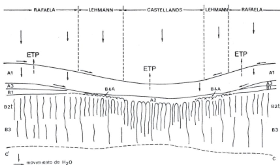
Figura 6.2. Microtoposecuencia de suelos hidro-halomórficos de la provincia de Santa Fe.
