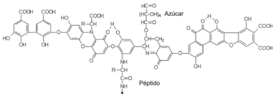
Figura 2.5. Estructura de ácidos húmicos propuesta por Stevenson (1994).
