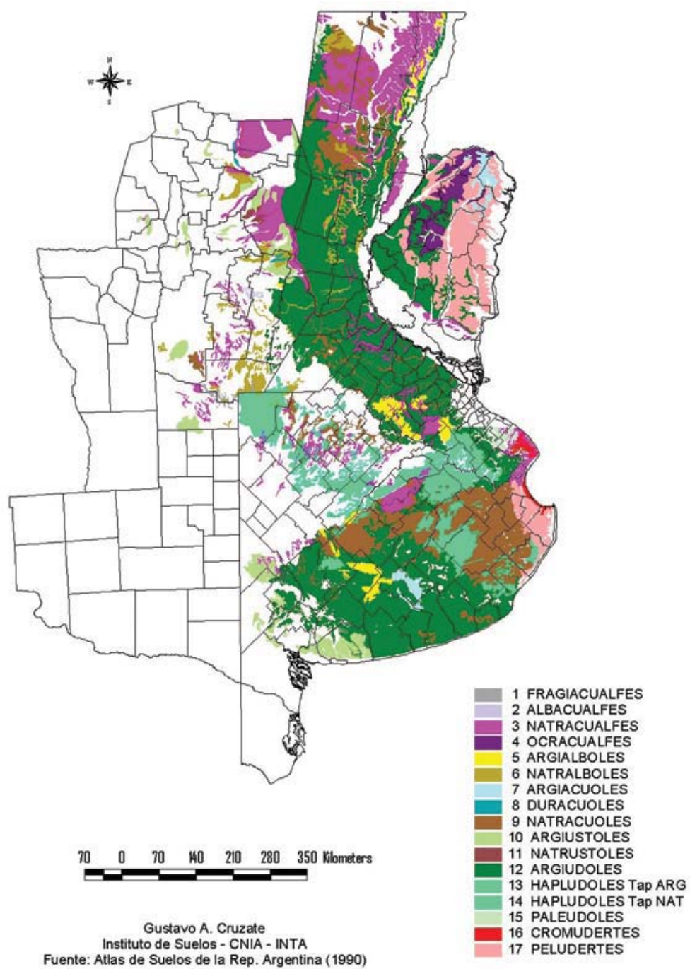
Figura 3.1. f) Grandes Grupos de suelos con ilimerización.
