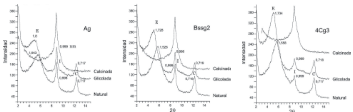
Figura 5.16. Registros difractométricos de un Acuert (Pedón 2, Tabla 5.6) de la Planicie costera del Río de la Plata provincia de Buenos Aires. Imbellone et al., 2006.
