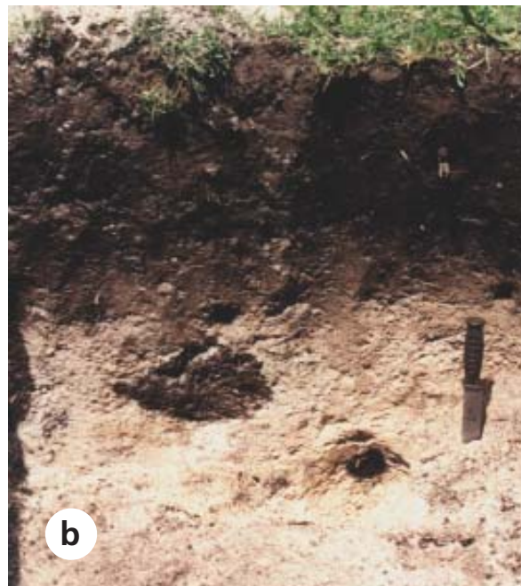
Figura 2.7. a) Perfil de la Serie Santa Isabel (Hapludol típico, INTA 1983) con evidencia de reciclado de materiales; crotovinas, actividades de la mesofauna mezclando materiales de diversos horizontes, deyecciones de lombrices. b) efecto de la mesofauna en Haprendoles.
