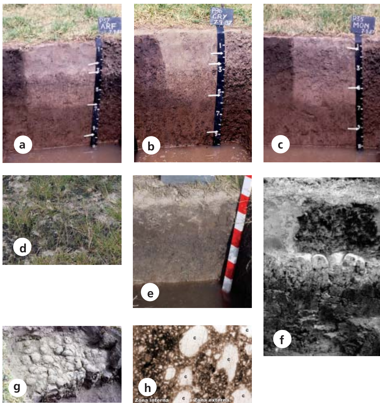
Figura 6.3. Perfiles de suelos representativos de los Bajos Submeridionales: a) Natralbol típico (Serie Arrufó), Natracuol típico (Serie Curupaytí), c) Natracualf típico (Serie Monigotes). Suelos afectados por sales de la Pampa Deprimida: d) encostramiento superficial en Natracualf, con presencia de Distichlis spp. y Nostoc spp. , e) Natracualf con humatos y fulvatos sódicos en agua freática, f) estructura columnar en Natracualf (Solonetz solodizado), Oliden, partido de La Plata, provincia de Buenos Aires, g) vista superior de la estructura columnar, h) sección delgada (sin analizador, 36X) de un corte longitudinal de una columna de suelo. Zona externa con macrocavidades (c), zona interna densa.
