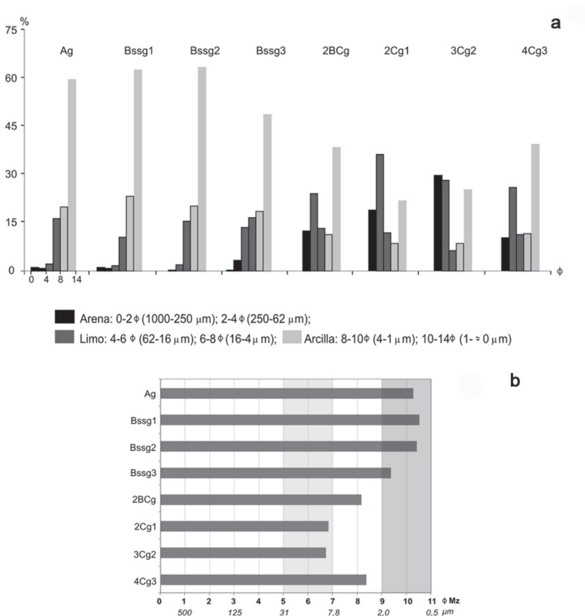
Figura 5.17. Distribución granulométrica de un Natracuert. Partido de Berazategui. a) Histograma, b) Media aritmética. Arena (1000-62μm, 0-4 φ) ; limo (62-4μm, 4-8φ); arcilla (4-1μm, 8-10φ); <1 μm valores inferidos a partir de la curva acumulativa. Imbellone y Mormeneo, información inédita.
