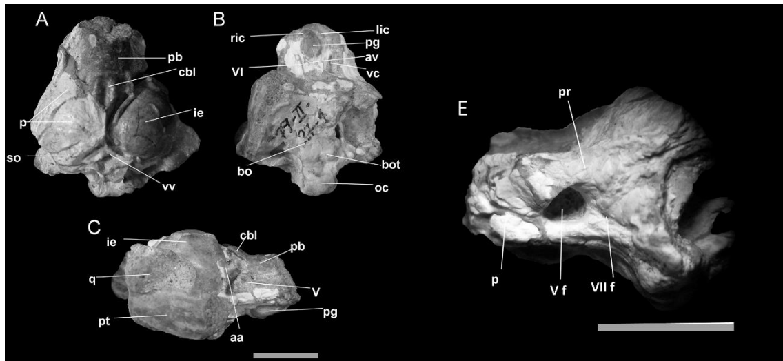
Figura 43. Cráneo de Dinilyisia patagonica , MLP 79-II-27-1. La barra de escala equivale a 10 mm. (A) Vista dorsal, (B) vista ventral, (C) vista lateral derecha y (D) vista lateral izquierda. Abreviaturas: aa, ampolla anterior; av, vasos aórticos; bo, basioccipital; bot, tubérculos basioccipitales; cbl, cerebelo; ie, oído interno; lic, carótida interna izquierda; oc, cóndilo occipital; p, parietal; pb, encéfalo posterior; pg, glándula pituitaria; pr, proótico; pt, pterigoides; q, cuadrado; ric, carótida interna derecha; so, supraoccipital; V, nervios trigémino; VI, abducen los nervios; vc, canal vidiano; Vf, foramen nervio trigémino; VII f, foramen nervio facial; vv, vasos vasculares.
