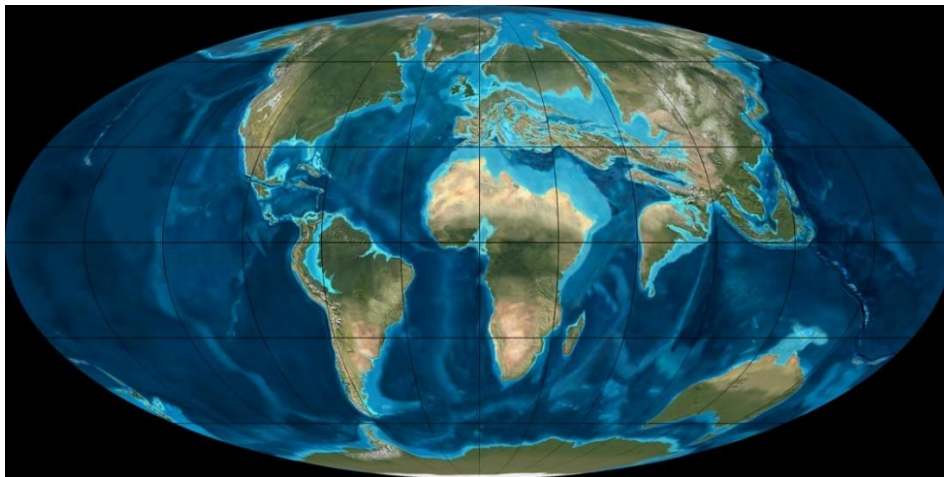
Figura 84: Eoceno. 50 millones de años. Tomado de http://jan.ucc.nau.edu/rcb7/mollglobe.html
