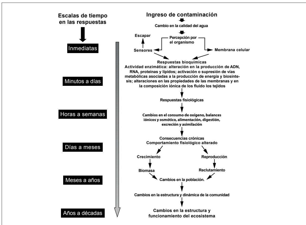
Figura 2: Sucesión de cambios esperados en la biota frente a una perturbación en un ecosistema acuáticos (modificado de Vernberg, & Vernberg, 1981).
