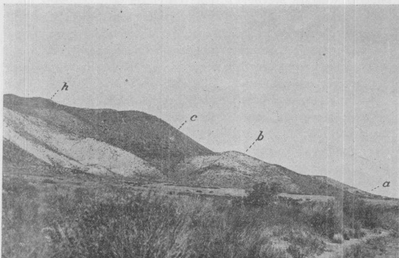
Fig. 3. — Carrin-curá. Ladera izquierda del valle. Sedimentos titonienses (Para las letras véase el perfil y el texto)
