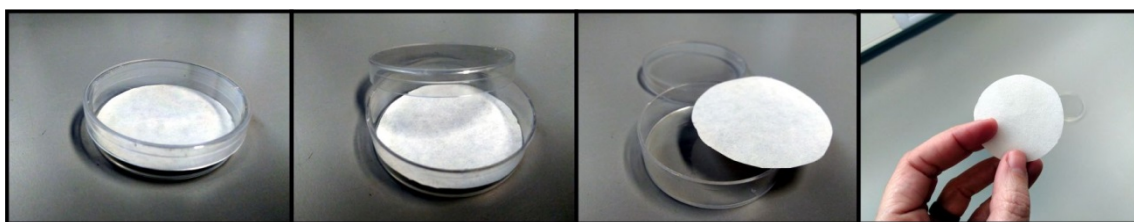
Fig. 3-7. Cápsula de Petri de 5,3 cm de diámetro y papel de filtro de 5 cm utilizados para el ensayo por exposición residual sobre papel de filtro (residuo seco).
