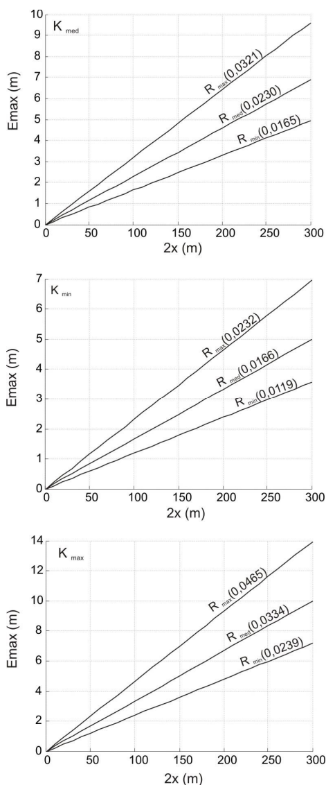
Figura 3. Estimación de la variación del espesor máximo ( E_{max} ) de las lentes de agua dulce en función del ancho del cordón de conchilla para valores de conductividades hidráulicas medias ( K_{med} ), mínimas ( K_{min} ) y máximas ( K_{max} ), y para valores de recarga media ( R_{med} ), mínima ( R_{min} ) y máxima ( R_{max} ). Entre paréntesis se indica el valor de las pendientes de las rectas.
