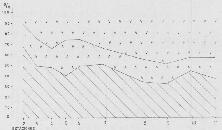
Fig. 6. — Litología total. Se representa con v a los granitos grises y con v invertida a los granitos rosados; las líneas oblicuas representan a las rocas no graníticas.
