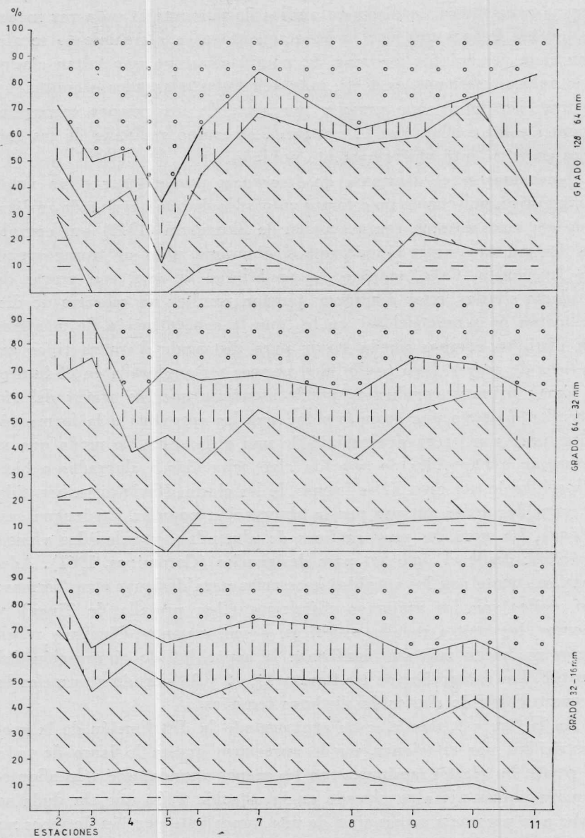
Fig. 10. --- Geometricidad según grados. Mismos símbolos que para la figura 9
