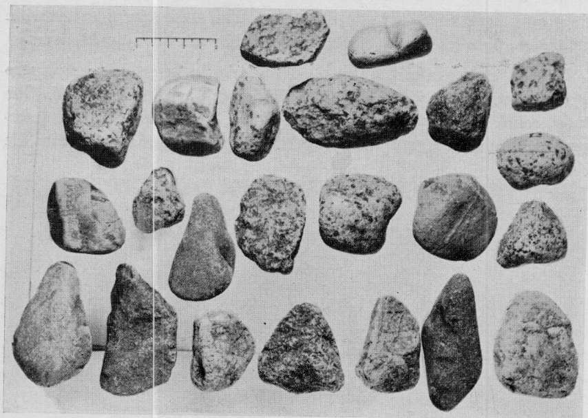
Fig. 12. — Clastos del grado 64-32 mm. Estación 4
