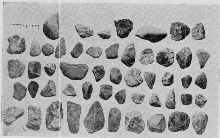
Fig. 13. — Clastos del grado 32-16 mm. Estación 4
