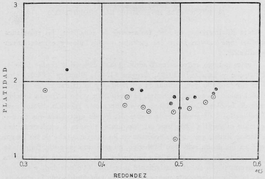
Fig. 22. — Relación entre redondez y platidad. Mismos símbolos que para la figura 21
