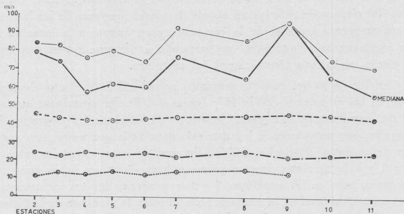
Fig. 5. — Diagrama de variación de mediana y medias. Línea entera : media del grado 128-64 mm ; línea cortada : media del grado 64-32 mm ; línea rayada y punteada : media del grado 32-16 mm ; línea punteada : media del grado 16-8 mm.
