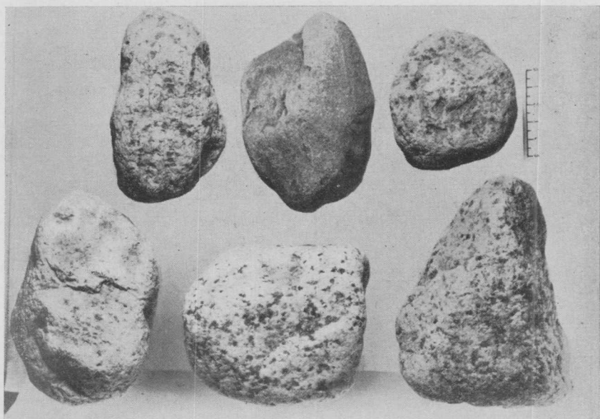
Fig. 11. — Clastos del grado 128-64 mm. Estación 4
