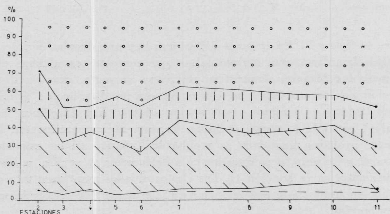
Fig. 14. — Geometricidad de clastos graníticos. Mismos símbolos que para las figuras 9 y 10
