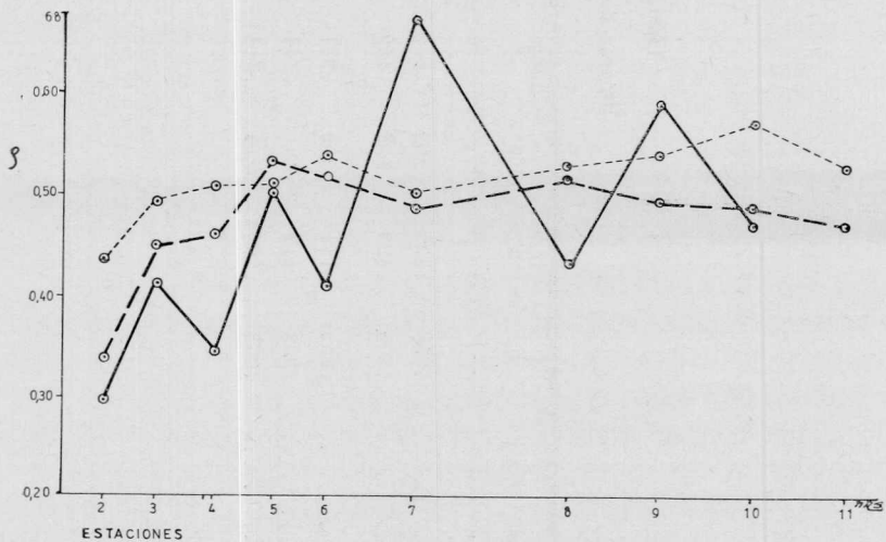
Fig. 20. — Redondez según grados. Línea entera : grado 128-64 mm ; línea cortada: grado 64-32 mm ; línea punteada : grado 32-16 mm
