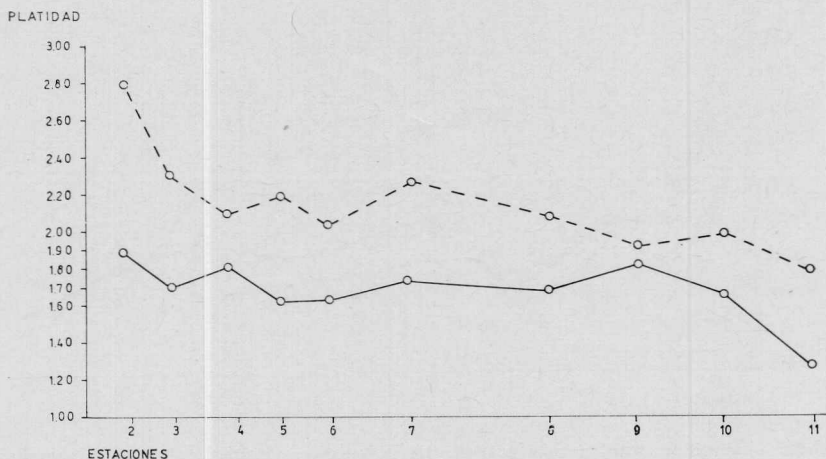
Fig. 16. — Platitude según litología. Línea entera : rocas graníticas ; línea cortada : rocas no graníticas
