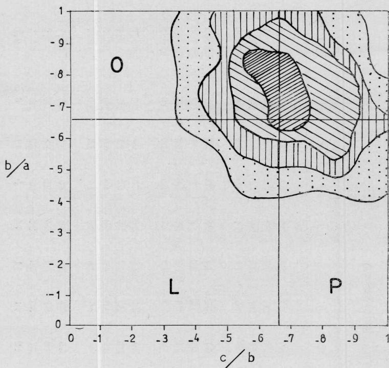
Fig. 8. — Diagrama de frecuencia de geometricidad. Contornos de 4 o/o, 3 o/o, 2 o/o y 1 o/o por área de 1 o/o. Total de 2300 clastos
