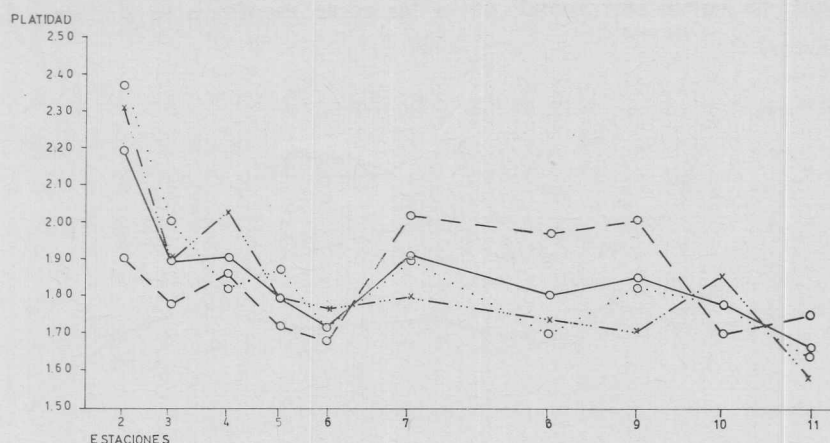
Fig. 15. — Platidad total y por grados. Línea entera : platidad total; línea cortada : grado 128-64 mm ; línea punteada : grado 64-32 mm y línea rayada y punteada : grado 32-16 mm.
