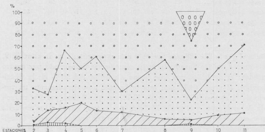
Fig. 4. — Granulometría de las gravas. Ovalos: grado 256-128 mm; círculos: grado 128-64 mm; puntos: grado 64-32 mm; rayas oblicuas: grado 32-16 mm; rayas verticales: grado 16-8 mm.
