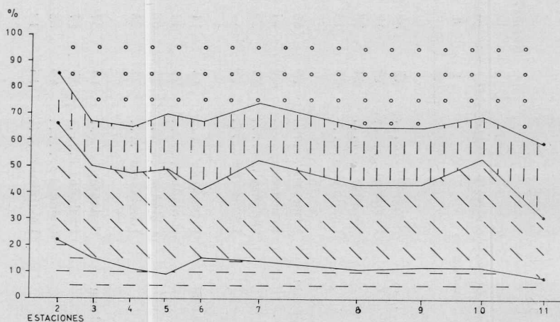
Fig. 9. — Geometricidad total. Círculos: clastos ecuanter; líneas verticales: clastos prolados; líneas diagonales: clastos oblados; líneas horizontales: clastos laminares.
