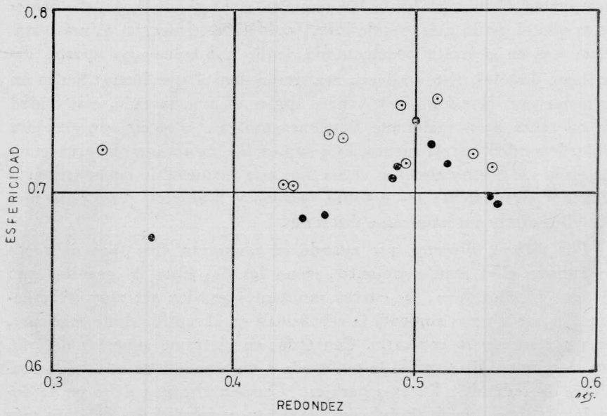
Fig. 21. — Relación entre redondez y esfericidad. Puntos llenos : valores totales de las gravas ; círculos blancos : valores de clastos graníticos
