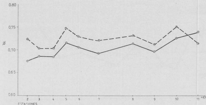
Fig. 17. — Curvas de esfericidad. Línea gruesa : esfericidad total ; línea cortada : esfericidad de clastos graníticos
