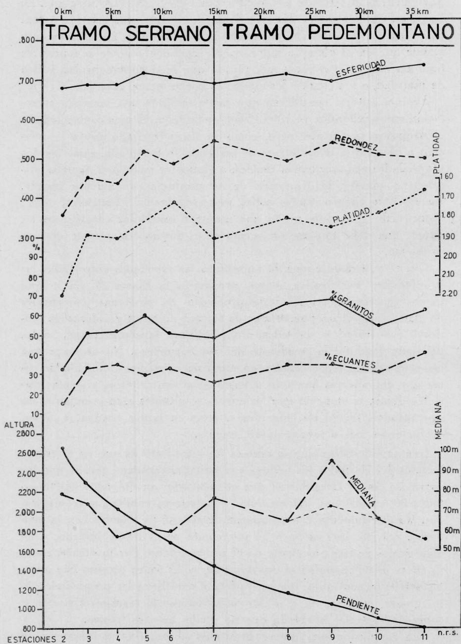
Fig. 23. — Diagrama del conjunto de propiedades sedimentológicas de las gravas y de pendiente del río Sarmiento
