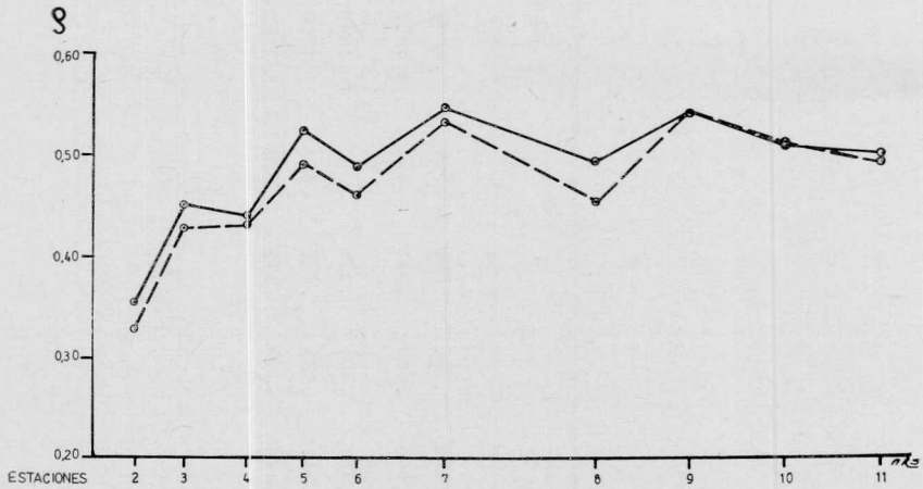
Fig. 19. — Curvas de redondez. Línea entera : redondez total ; línea cortada redondez de elastos graníticos
