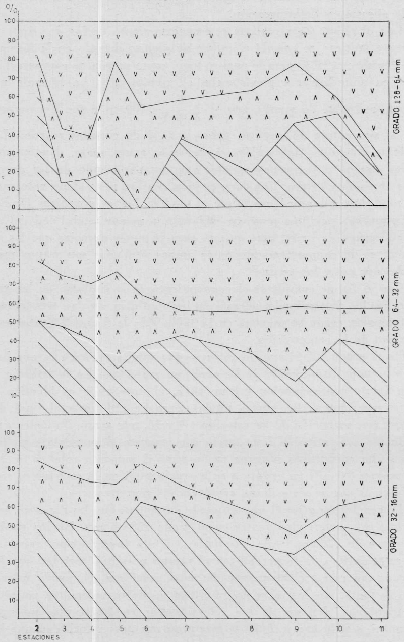
Fig. 7. Litología según grados. Mismos símbolos que para la figura 6
