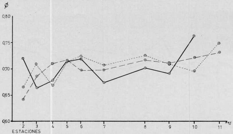
Fig. 18. — Esfericidad según grados. Línea entera : grado 128-64 mm ; línea cortada : grado 64-32 mm ; línea punteada : grado 32-16 mm
