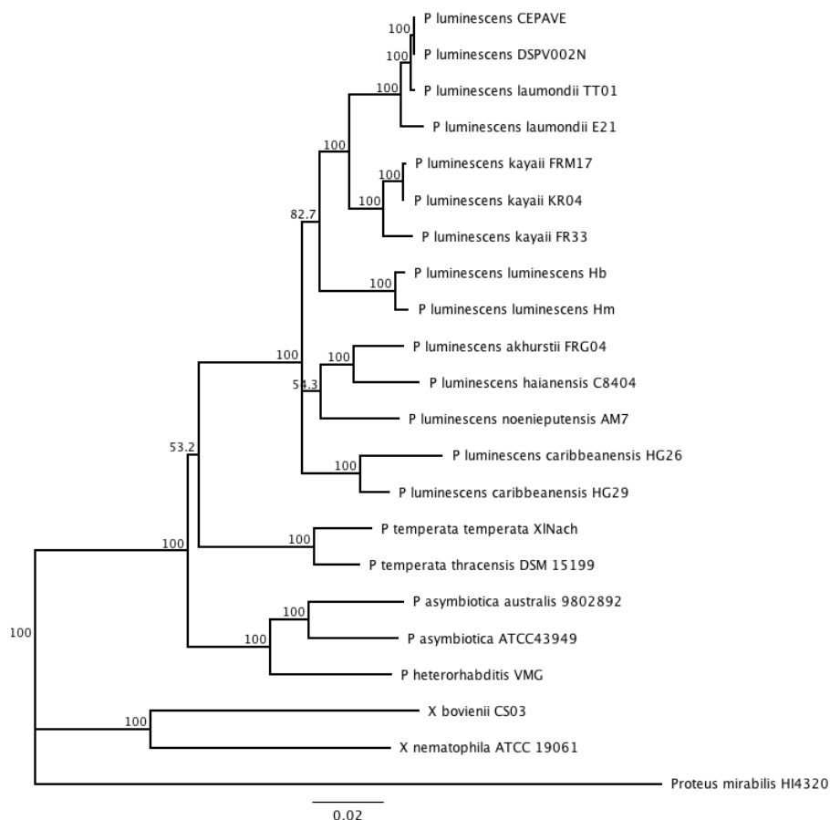
Figura 1.7. Concatenado de cinco genes ( recA , gyrB , dnaN , gltX e infB ) (Ferreira et al., 2013) que representan 3,800 nucleótidos en total, utilizando el método Neighbor-Joining implementado en Geneious R11 (Drummond et al. 2018). Se utilizó un remuestreo de arranque de 1000 y se exhibieron valores de soporte de consenso superiores al 50% en cada nodo.
