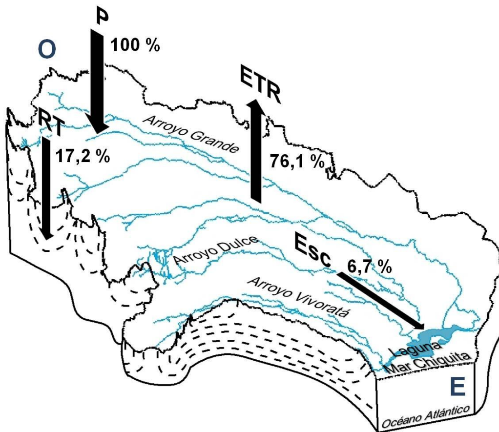
Figura 7.8. Balance hídrico del sector meridional de la cuenca de la laguna Mar Chiquita. Las líneas discontinuas representan flujos de agua subterránea locales y regionales ( P : precipitación, ETR : evapotranspiración real, RT : recarga potencial o de tránsito, Esc : escurrimiento superficial)
