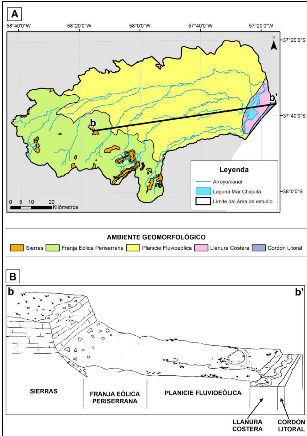
Figura 5.2.A. Mapa geomorfológico del área de estudio (extraído y modificado de Martínez et al. , 2001), B. Block diagrama mostrando los ambientes geomorfológicos presentes en la sección b-b' (extraído y modificado de Martínez, 2001 b)
