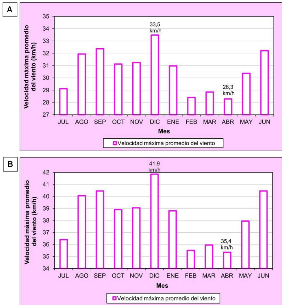
Figura 3.23. Velocidad máxima promedio mensual del viento en la Estación Mar del Plata Aeropuerto (1971-1990) registrada a: A. 2 m de altura, B. 10 m de altura
