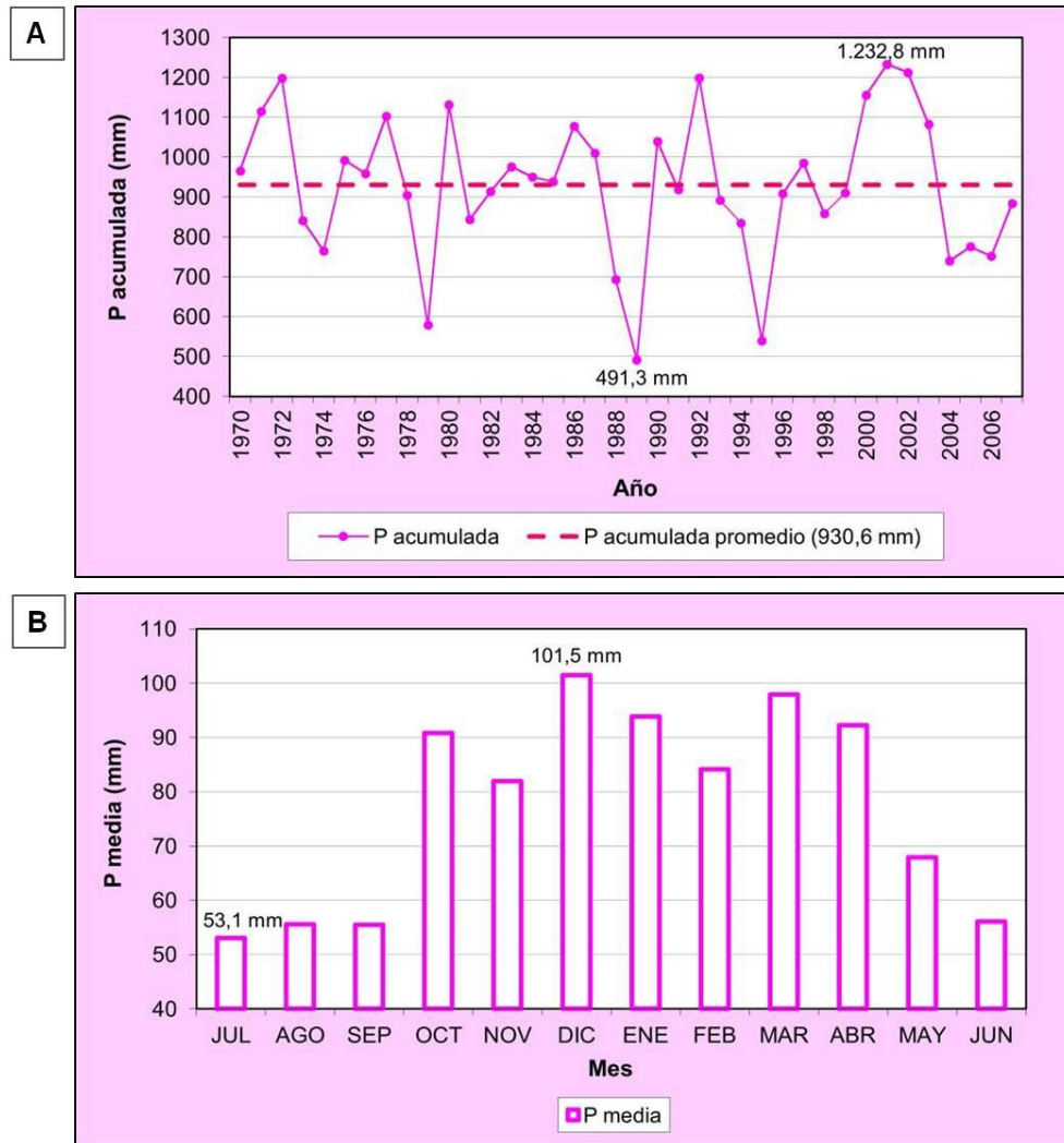
Figura 3.19. Precipitación (P; mm) en la Estación Mar del Plata Aeropuerto (1970-2007): A. Acumulada anual, B. Media mensual
