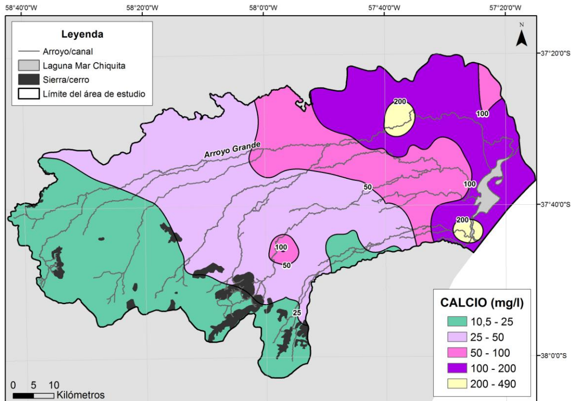
Figura 8.12. Distribución espacial del catión calcio (mg/l) en el agua subterránea
