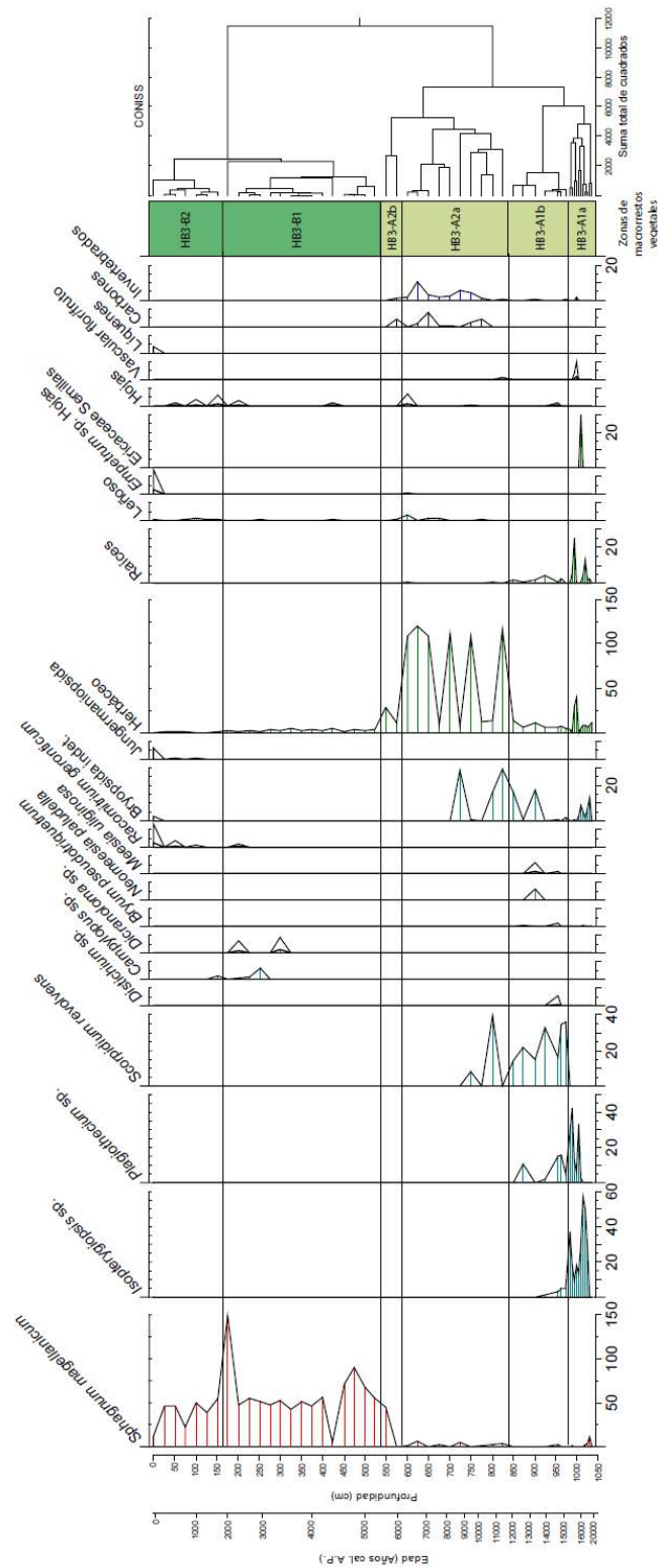
Fig. 22. Diagrama de concentración (n° de macrorestos por 5 cm 3 ) detallado del testigo Harberton 3 incluyendo especies, géneros y morfotipos de briofitas y plantas vasculares.
