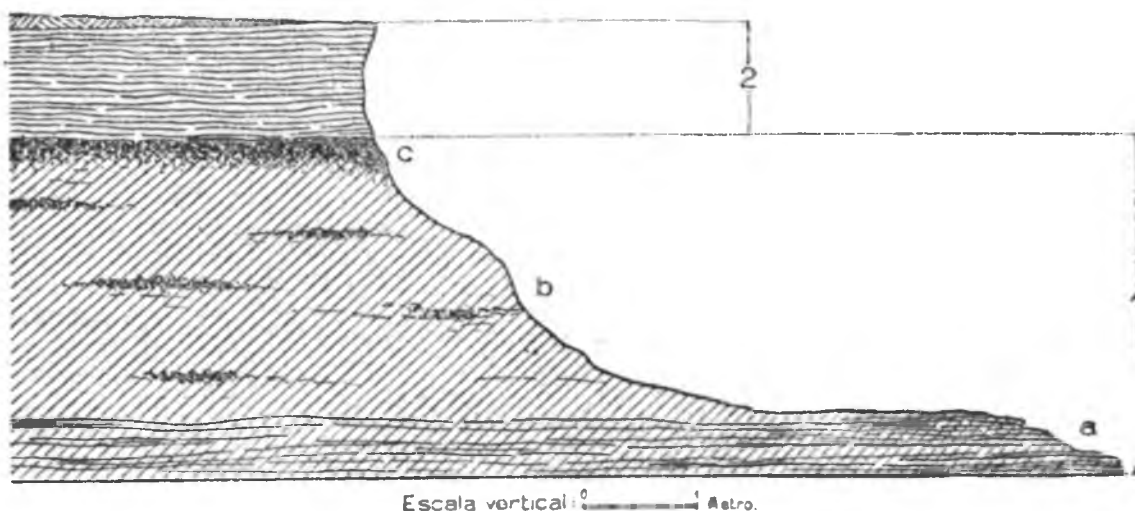
Fig. 6. — Barranca del río Salado, aproximadamente a la altura de Colonia Videla. 1, lujanense: a, limos pardos y verde grisáceos, arcillosos, con intercalaciones de capas lenticulares, extendidas, delgadas e imbricadas, de tosca, a veces travertinosa, conteniendo, en partes, numerosos restos de Corbícula , Diplodon , Anodontidis (fase fluvial); b, limo arcilloso pardo, sin estratificación, con pequeñas tosquillas calcáreas ramificadas, esparcidas, con restos de Platemys y Mastodon ; c, zona superior del precedente con tosquillas calcáreas numerosas y confluentes (fase palustre). 2, platense, limos grises, en partes con Planorbis peregrinus , Littoridina Parchappi y Ampullaria canaliculata (original de Joaquín Frenguelli).
