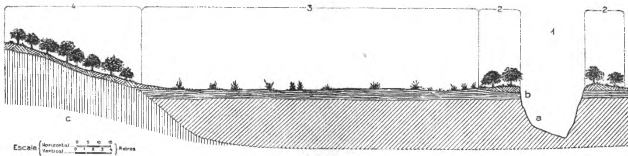
Fig. 5. — Perfil transversal de la margen izquierda del valle del río Salado, aproximadamente a la altura de la Colonia Videla. a-b, post-pampeano (véanse detalles en la figura siguiente); c, pampeano: 1, cauce actual del Salado, 2, bordes terraplenados del río con galería de algarrobos, espinillos, curupí y sina-sina, 3, terraza baja post-pampeana, inundable durante las grandes crecidas del río, con pradera de Solanáceas, Ciperáceas y Gramináceas, entre las cuales sobresalen matas de Gynerium argenteum , alternadas con almarjales, 4, terraza pampeana con talud suavemente inclinado, fuera ya del alcance de las aguas del río y revestida de monte relativamente denso: quebrachos, tala, chañar, algarrobos, espinillos, aromito, ñandubay, etc. (original de Joaquín Frenguelli).
