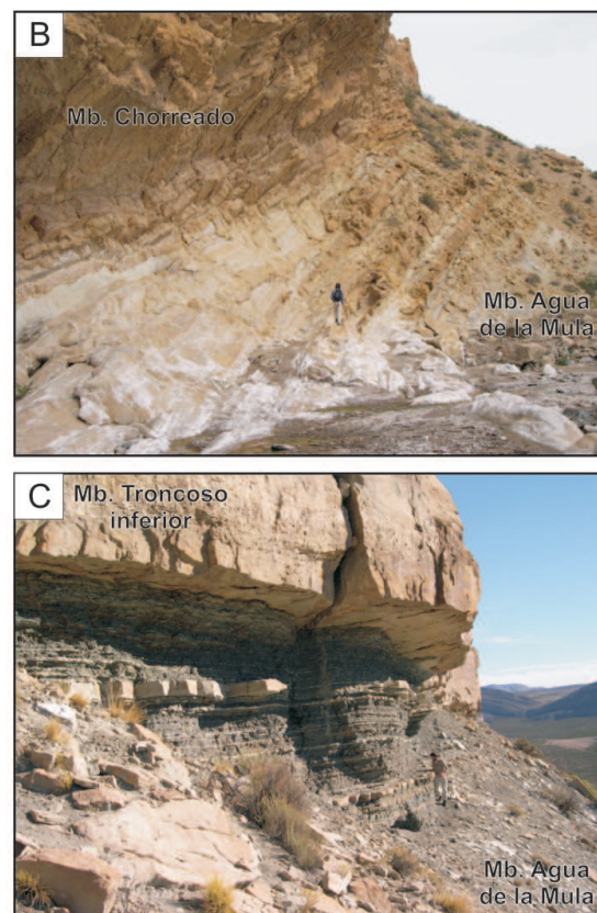
Figura 7: A) Perfiles representativos de la parte superior del Mb. Agua de la Mula (tomado de Veiga et al. 2005) en los que se aprecian sus relaciones estratigráficas con unidades suprayacentes, las facies constitutivas y los principales atributos sedimentarios. B) Vista de los depósitos del tope de la Formación Agrio en el área de El Portón. Nótese la disposición granocreciente de los cuerpos sedimentarios. C) Vista de detalle del tope de la Formación Agrio (Mb. Agua de la Mula) en la región de Pampa de Tril. Se aprecia el desarrollo de sucesiones heterolíticas con intercalaciones de areniscas con estratificación entrecruzada.
