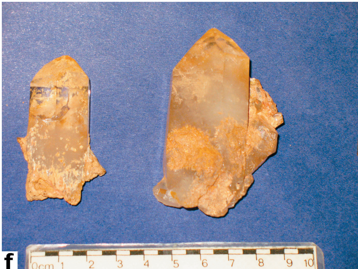
Figura 22f. Megacrystales de cuarzo piramidales, encontrados en dolomías (depósitos algales laminares) meteorizadas (Facies Carbonáticas-Siliciclásticas) de la Formación Villa Mónica, Estancia La Siempre Verde, Sierra La Juanita.
