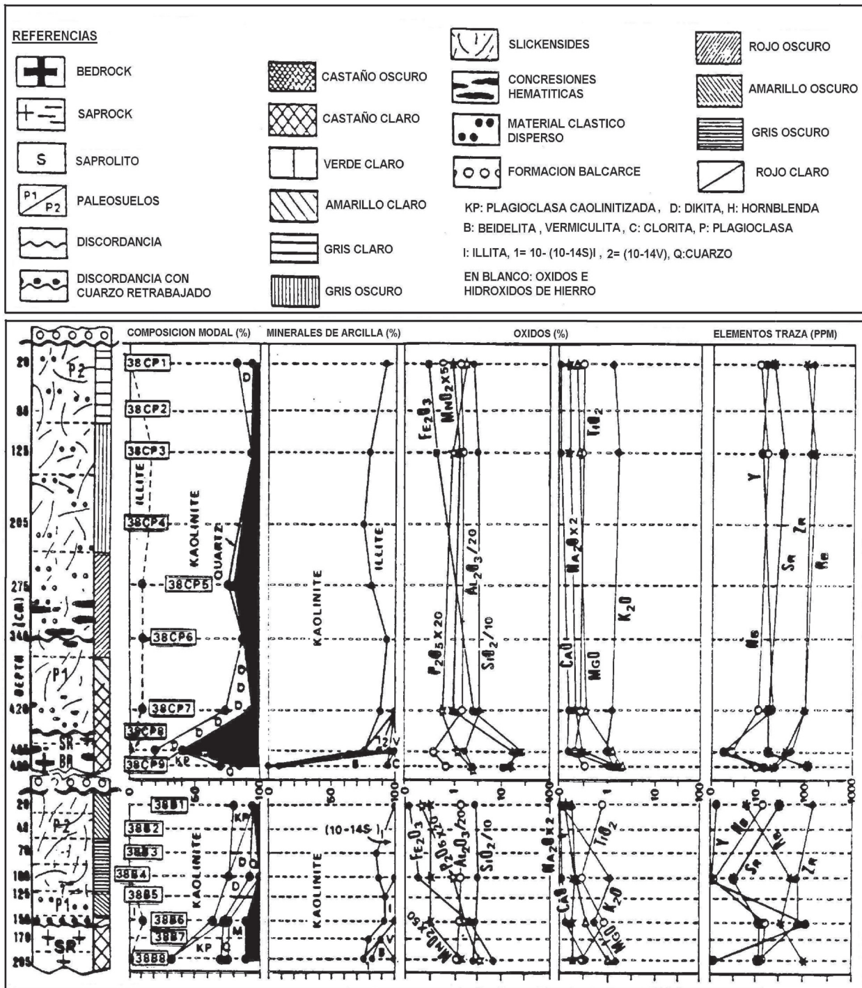
Figura 12. Constante 10. Dos perfiles (38CP y 38B) de detalle de la composición modal de las rocas del basamento alterado y los paleosuelos I y II, mineralogía de arcilla, porcentaje en peso de óxidos y elementos traza (Iñíguez et al. 1990).
