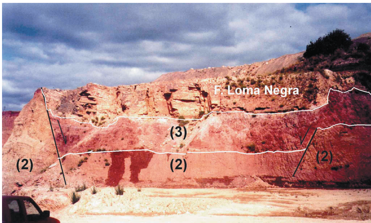
Figura 37. Formación Olavarría, cantera Dos Hermanos, Sierras Bayas. Pelitas ocreas (2); pelitas rojizas (3), cubierta en discordancia por la Formación Loma Negra. Las flechas indican el movimiento relativo de los bloques.
