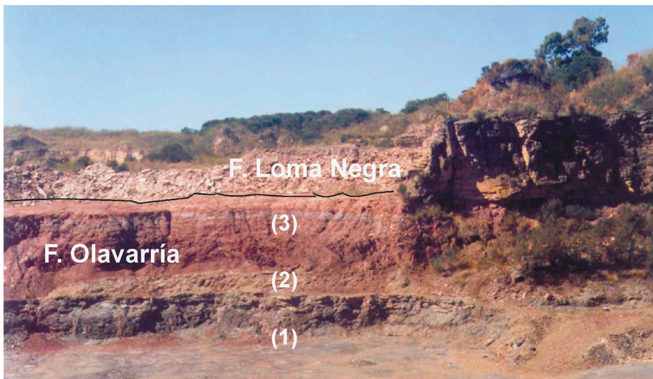
Figura 36. Formación Olavarría, Cantera Cruz Pavone, Sierras Bayas. Pelitas grises (1); pelitas ocreas (2); pelitas rojizas (3). Por encima, y en discordancia, se encuentra la Formación Loma Negra.
