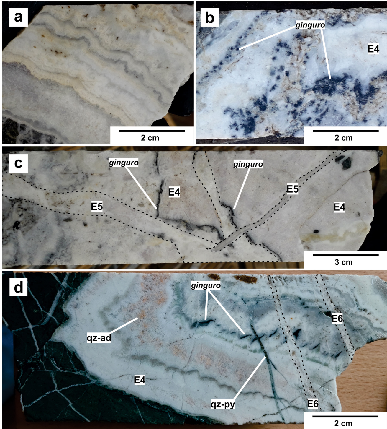
Figura 12. Fotografías de muestras de testigos de corona de perforaciones de la Veta 49. a) Bandeados coloformes silíceos del E4 (profundidad 168 m). b) Bandeados coloformes silíceos del E4, con ginguros moteados (profundidad 243 m). c) Sílice y carbonato masivos con ginguros del E4, interceptado por vetillas de sílice blanca masiva e incolora crustiforme del E5 (profundidad 142 m). d) Bandeados coloformes silíceos con adularia y escasos ginguros con deformación sigmoidal del E4, interceptados por vetillas de cuarzo y pirita del E5, además de vetillas de carbonato masivo del E6 (profundidad 296 m). Qz: cuarzo; Py: pirita; Ad: adularia.
