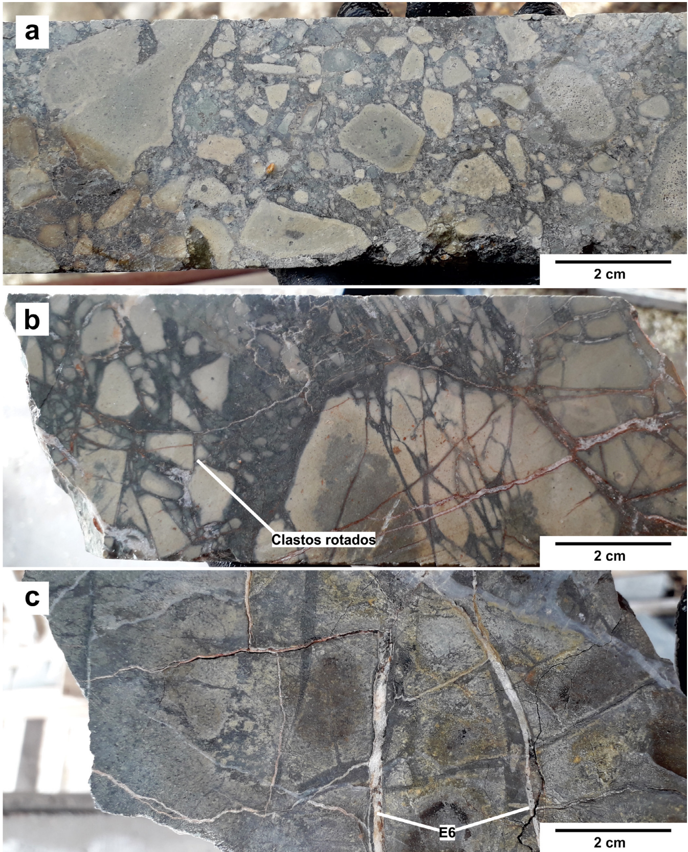
Figura 8. Fotografías de muestras de testigos de corona de perforaciones del sector de Veta 49. a) Brecha tectónica-hidrotermal del E1, con clastos subredondados de roca de caja y matriz de clorita-esmectita-pirita. b) Brecha tectónica-hidrotermal del E1, con clastos subangulosos a subredondados de roca de caja, a veces rotados. c) Brecha hidrotermal del E1, con fábrica en rompecabezas y vetillas del E6.
