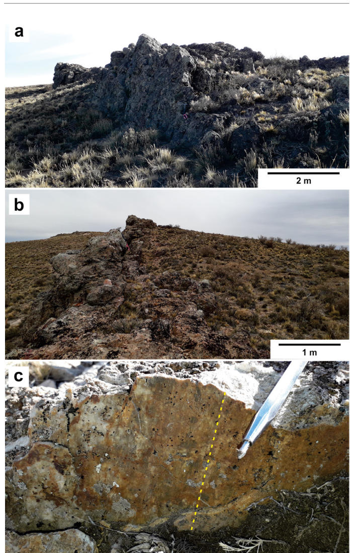
Figura 2. a y b) Fotografías de afloramientos de la Veta 49. c) Estrías de falla silicificadas en la Veta 49, resaltadas en línea punteada amarilla.
