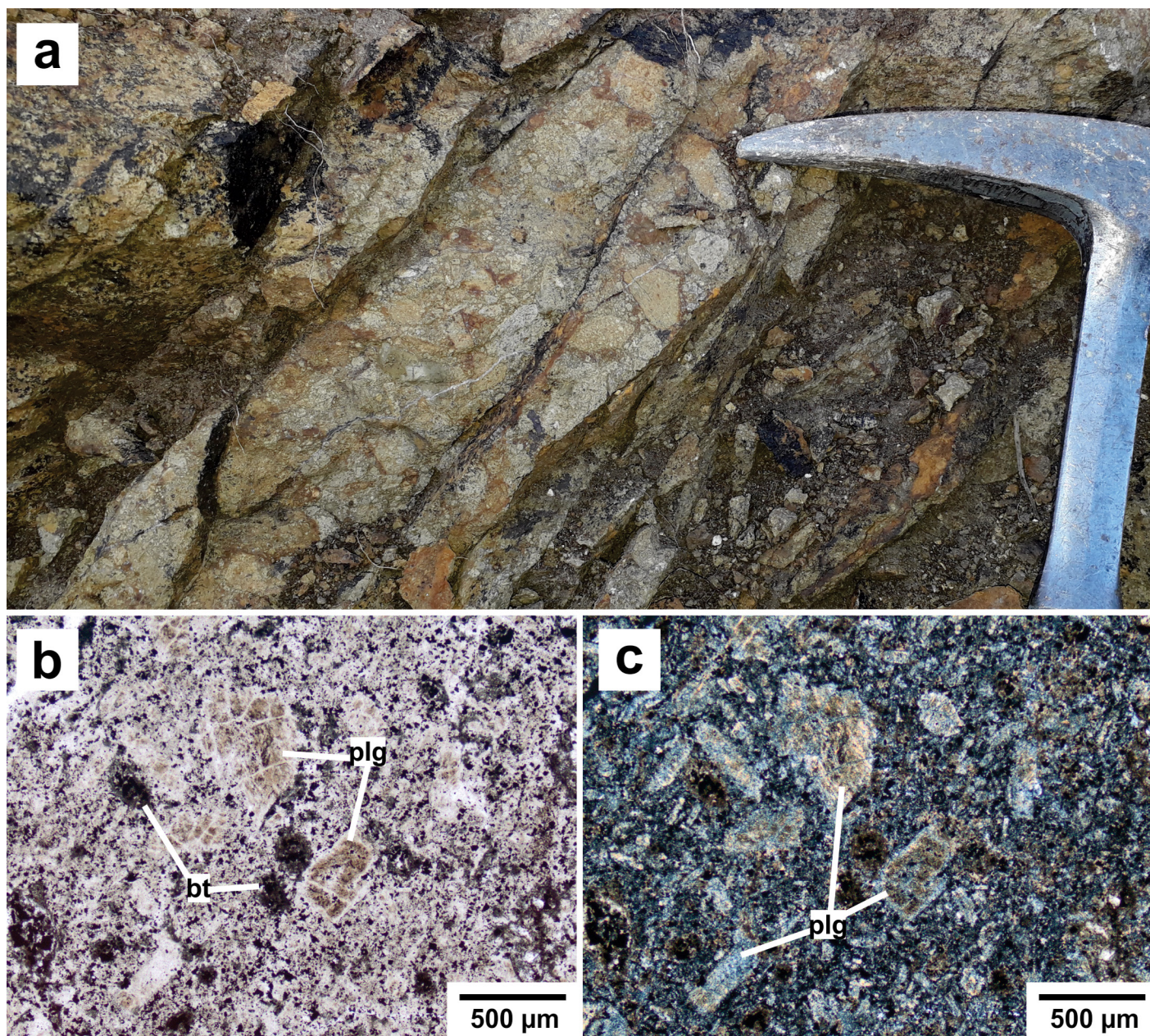
Figura 3. a) Afloramiento de autobrecha andesítica de la Formación Taquetrén. b y c) Micrografías de la autobrecha andesítica vista bajo nicols paralelos (B) y cruzados (C), donde se observan fenocristales de plagioclasa alterados a illita y de biotita reemplazados por clorita y pirita. Plg: plagioclasa; Bt: Biotita.
