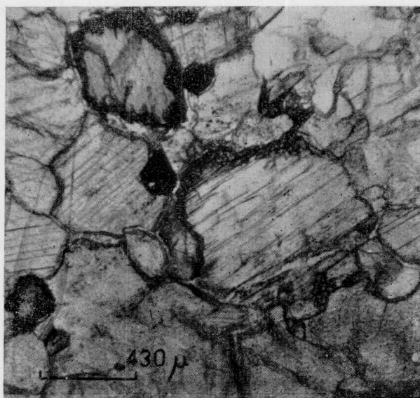
1. A la derecha, cristal de piroxeno rodeado por anillo de reacción (anfíbol) en una matriz de calcita. A la izquierda, cristal de escapolita con borde de reacción (epidoto). 2. Parte inferior, cristal de escapolita con borde de reacción en la parte superior del grano (epidoto). Parte superior foto, cristal de piroxeno, (ferrosalita) con borde de reacción (anfíbol).
