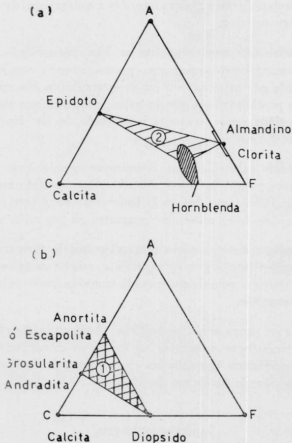
Fig. 11. — Diagramas Acf para mostrar posibles campos de estabilidad para las asociaciones minerales separadas como : (1). Piroxeno-escapolita- plagioclasa-granate-cuarzo; (2). Epidoto hornblenda-clorita-calcita-cuarzo-(granate) ; (a). Facie de Equistos verdes-Subfacie Cuarzo-albita-epidoto-almandino ; (b). Facie de Anfibolitas almandinicas-Subfacie : Sill-ortoc-almandino ; (a). Según Turner y Verhoogen. (1960) ; (b). Según Winkler. (1965)
