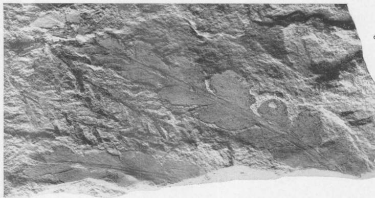
Dicroidium remotum Szajn. sp. Ejemplar nº 10.682 (a su izquierda la porción distal de una rama de Diplasiophyllum acutum Walk. sp.) ; 2, Ejemplar nº 10.699 ; 3, Ejemplar nº 10.680. Tamaño natural
