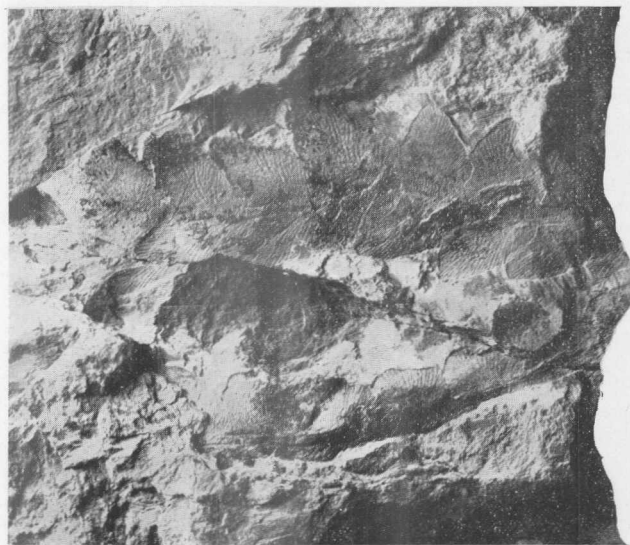
Dicrotidium remotum Szajn. sp. 1, Ejemplar nº 10.688, en tamaño natural; 2, Porción del mismo ejemplar ampliada \times 3 aproxim.
