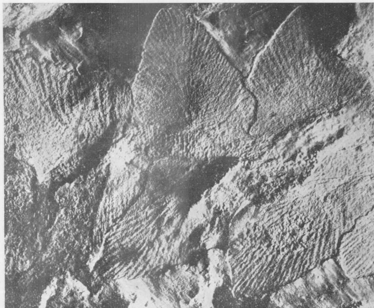
Dicrotidium remotum Szajn. sp. 1, Ejemplar nº 10.688, en tamaño natural; 2, Porción del mismo ejemplar ampliada \times 3 aproxim.
