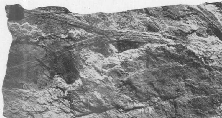
Dicroidium venotum Szajn. sp. 1, Ejemplar n° 10.683; 2, Ejemplar n° 10.684; 3, Ejemplar n° 10.685. Tamaño natural
