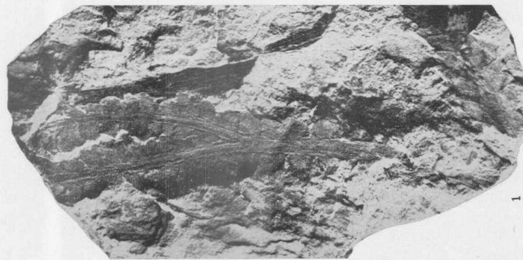
Dicroidium venotum Szajn. sp. 1, Ejemplar n° 10.683; 2, Ejemplar n° 10.684; 3, Ejemplar n° 10.685. Tamaño natural
