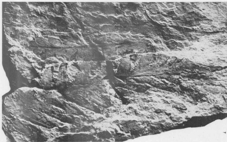
Dicroidium remotum Szajn. sp. Ejemplar nº 10.682 (a su izquierda la porción distal de una rama de Diplasiophyllum acutum Walk. sp.) ; 2, Ejemplar nº 10.699 ; 3, Ejemplar nº 10.680. Tamaño natural
