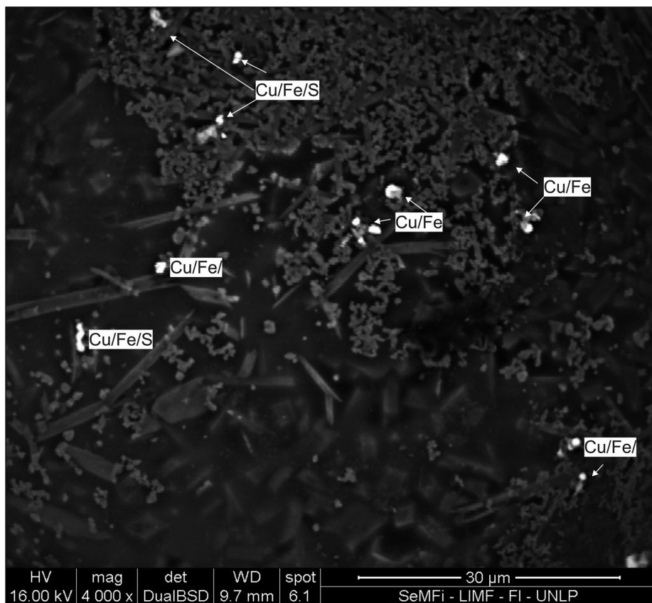
Figura 7. Escoria con glóbulos de \text{CuFeS} y \text{CuFe} . Imagen ESEM con electrones retrodifundidos de la M1. Slag with \text{CuFeS} and \text{CuFe} globules. ESEM Image with backscattered electrons of M1.
