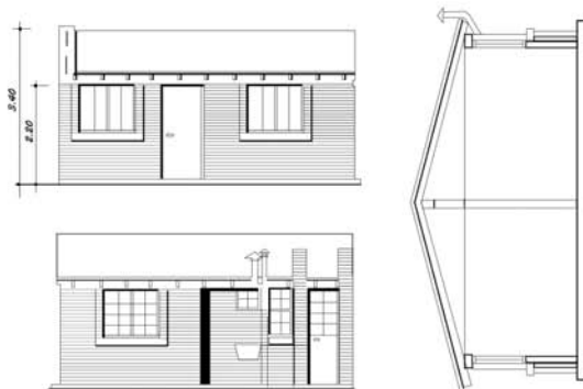
Planos de los "Chalecitos de los tobas"
