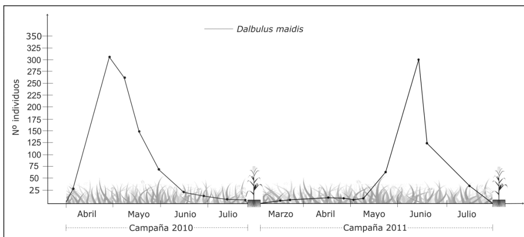
Fig. 2. Fluctuación poblacional de D. maidis en la región (ChSH) en la maleza asociada al maíz, durante los períodos otoño-invierno 2010 y 2011.
