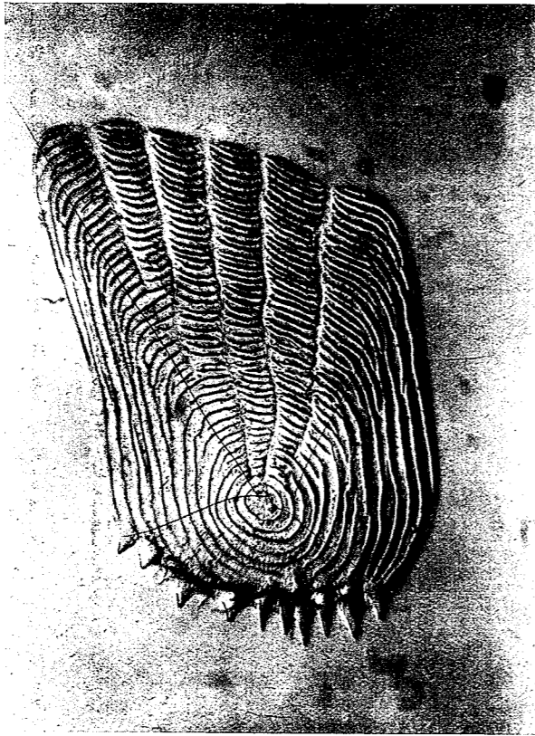
Fig. 6. — Escama de Cynoscion striatus (pescadilla) en la que se nota una marca de crecimiento, pero aun no se ha formado un anillo. Corresponde a un ejemplar de 75 mm. de longitud.
