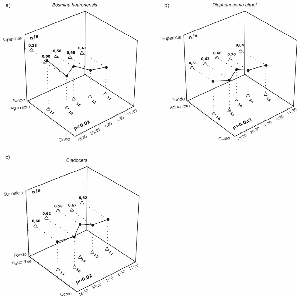
Figura 4. Variación de las respectivas posiciones medias horizontales en la transecta desde la costa hacia el centro de la laguna (números sobre el plano horizontal) y las medias verticales entre superficie y fondo (números sobre el plano vertical) en función del tiempo de Bosmina huaronensis , Diaphanosoma birgei y los cladóceros totales (en el plano correspondiente al posicionamiento se indica la significancia del análisis de ANOVA efectuado). Las distancias se expresan en metros.
