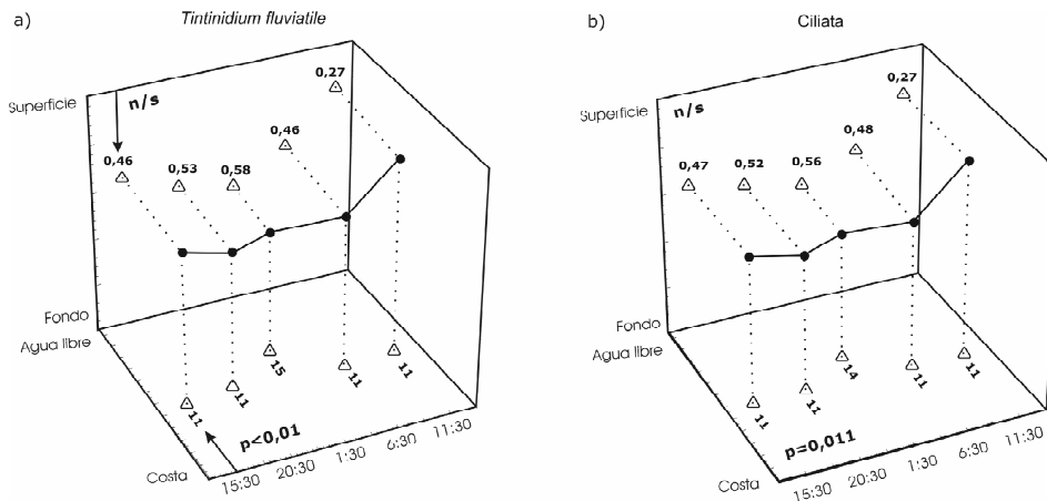
Figura 2. Variación de las posiciones medias horizontales en la transecta desde la costa hacia el centro de la laguna (números sobre el plano horizontal) y las medias verticales entre superficie y fondo (números sobre el plano vertical) en función del tiempo de la densidad de Tintinnidium fluviatile y el total de los ciliados (en el plano correspondiente al posicionamiento se indica la significancia del análisis de ANOVA efectuado). Las distancias se expresan en metros.
