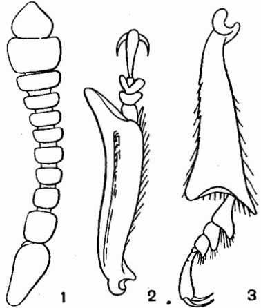
1. antena; 2. tibia y tarso anterior; 3. ídem posterior
